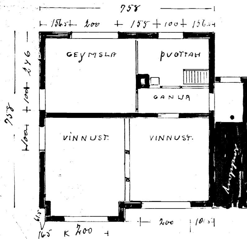
KJALLARI
