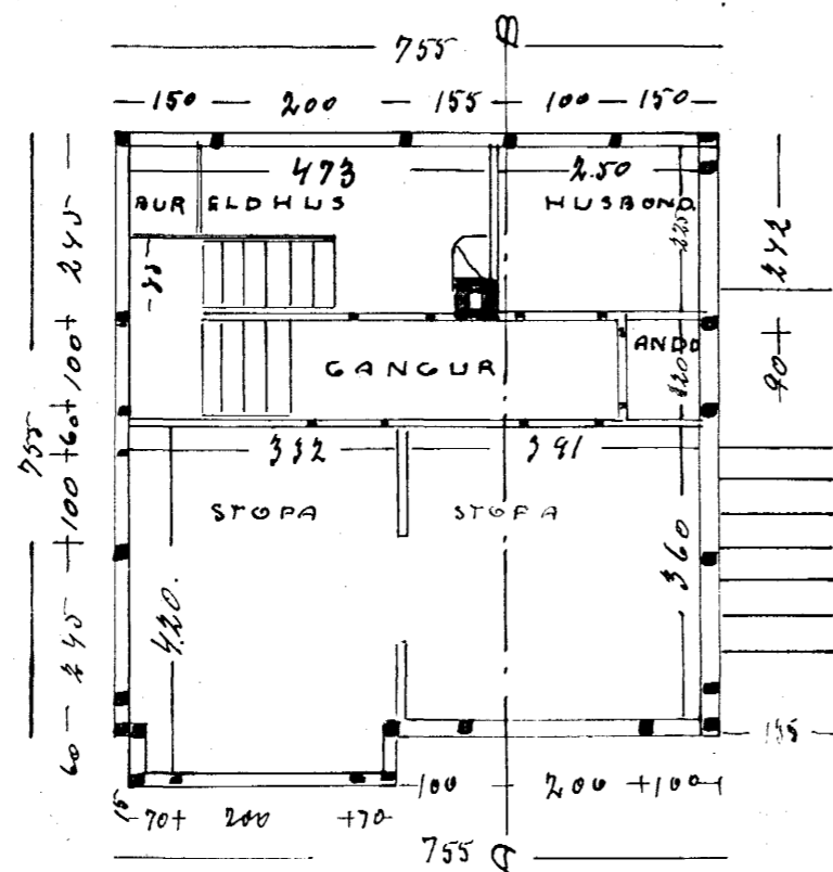
STOFUHLIÐ
