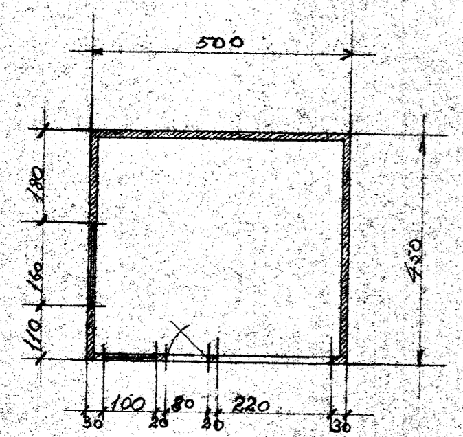
GRUNNMYND
