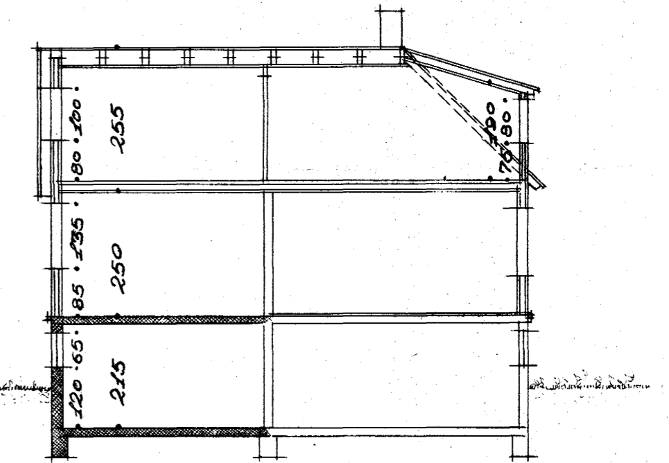
Sneiðing
