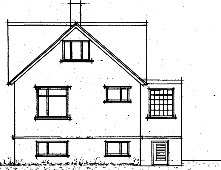
Vestur
