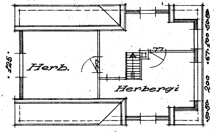
Rishæð
