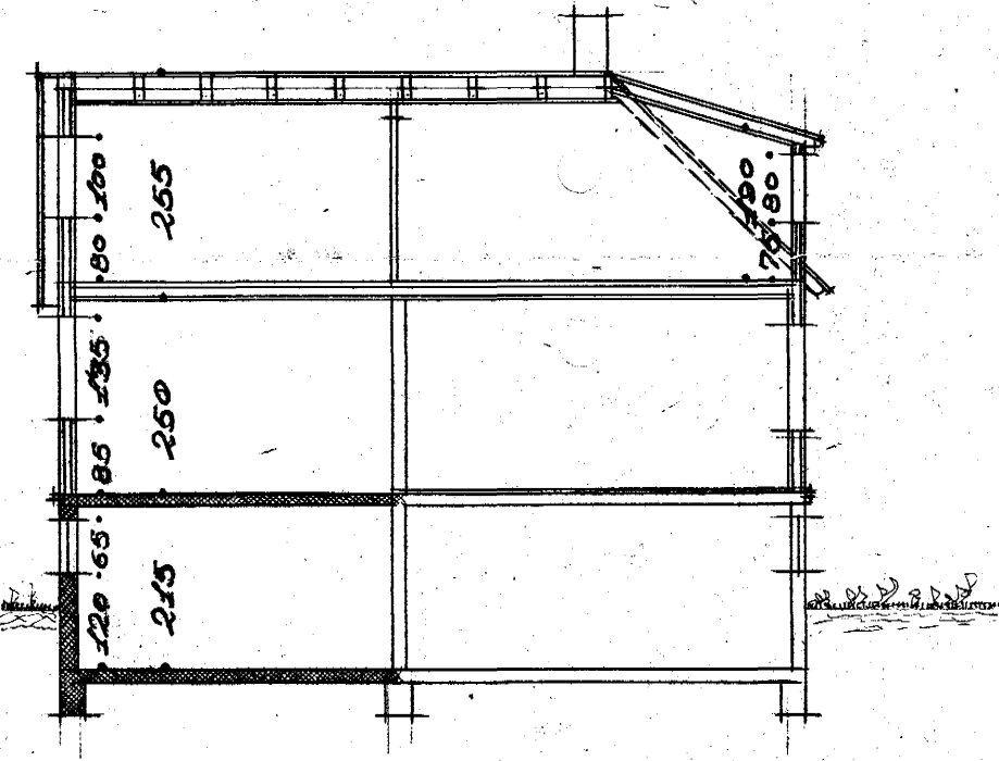
Sneiðing
