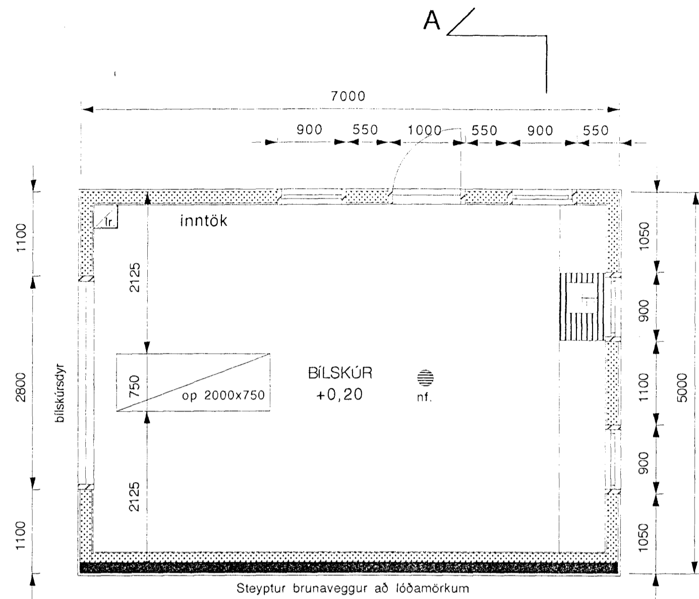
grunnmynd bilskúrs 1:50
