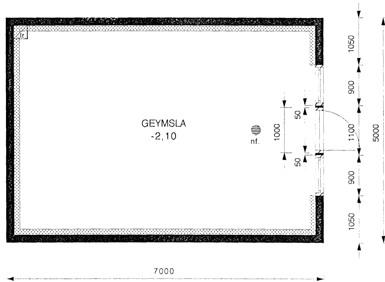
grunnmynd kjallara 1:50
