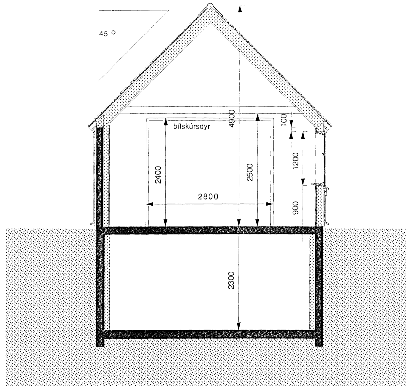
snið 1:50
