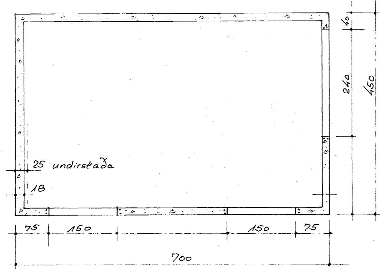
Grunnmynd 1:50
