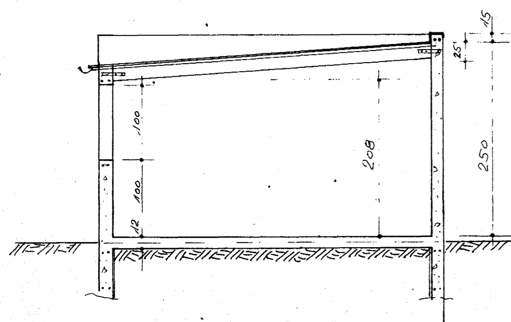
Snið 1:50
