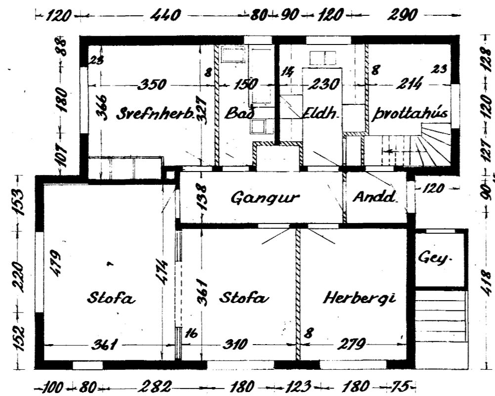
1. hæð
