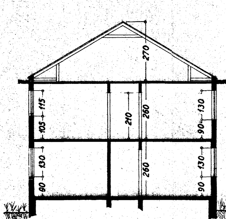
Sníð A-A
