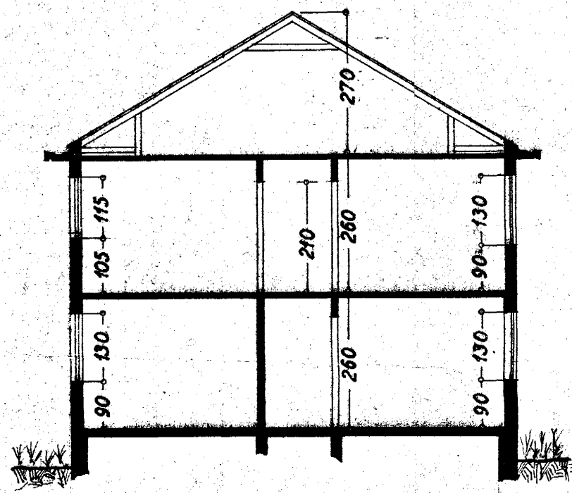
Snit A-A
