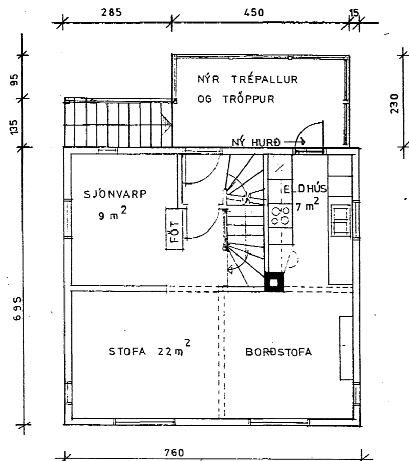
GRUNNMYND AÐALHÆÐAR 1:100
