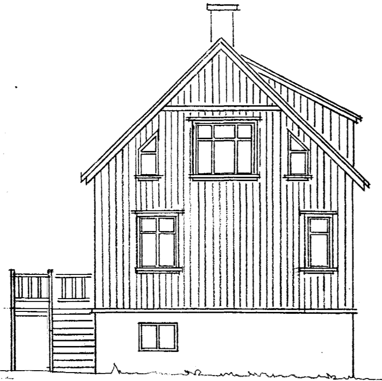
VESTUR 1:100
