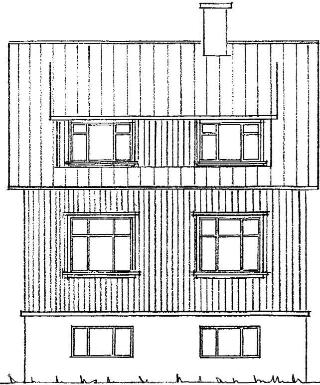
SUDUR 1:100
