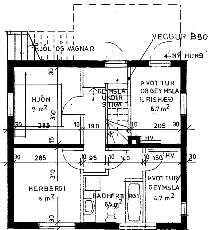
GRUNNMYND KJALLARA 1:100
