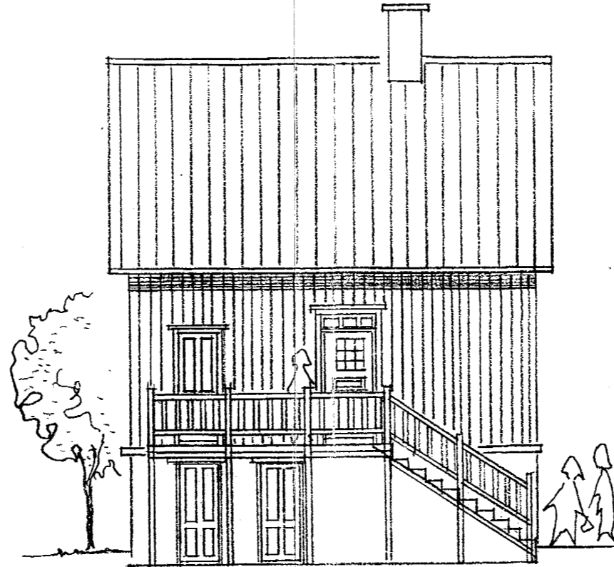
NORÐUR 1:100
