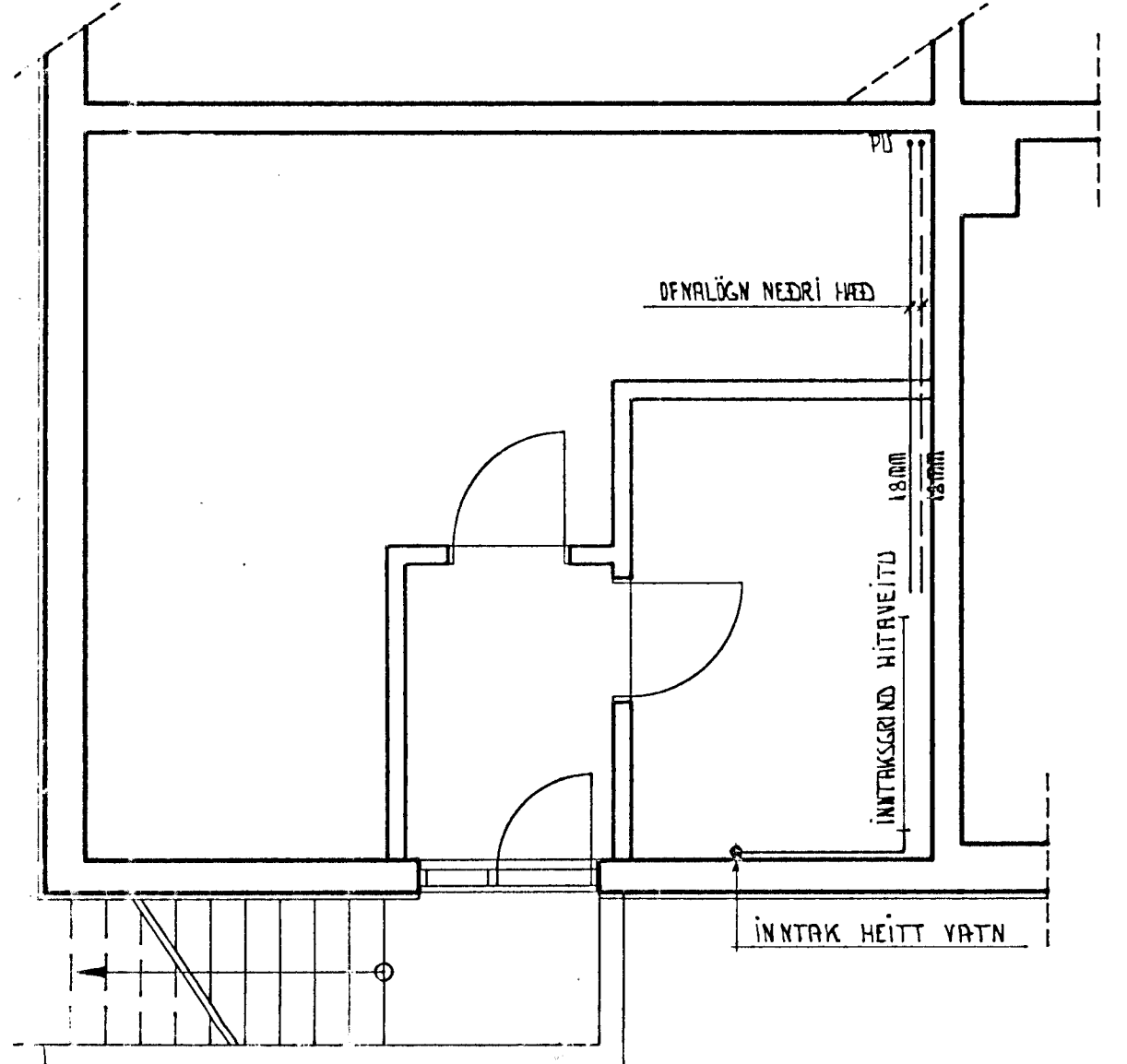
GRUNNMYND KJALLARI 1:50
