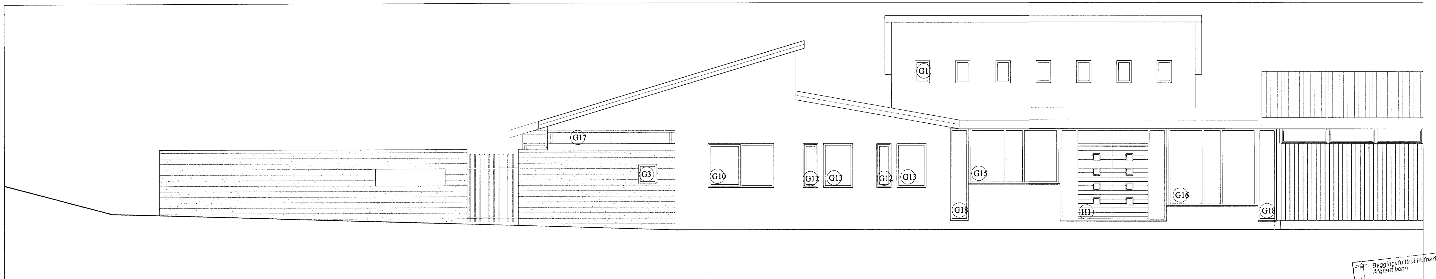
Útlit norður
