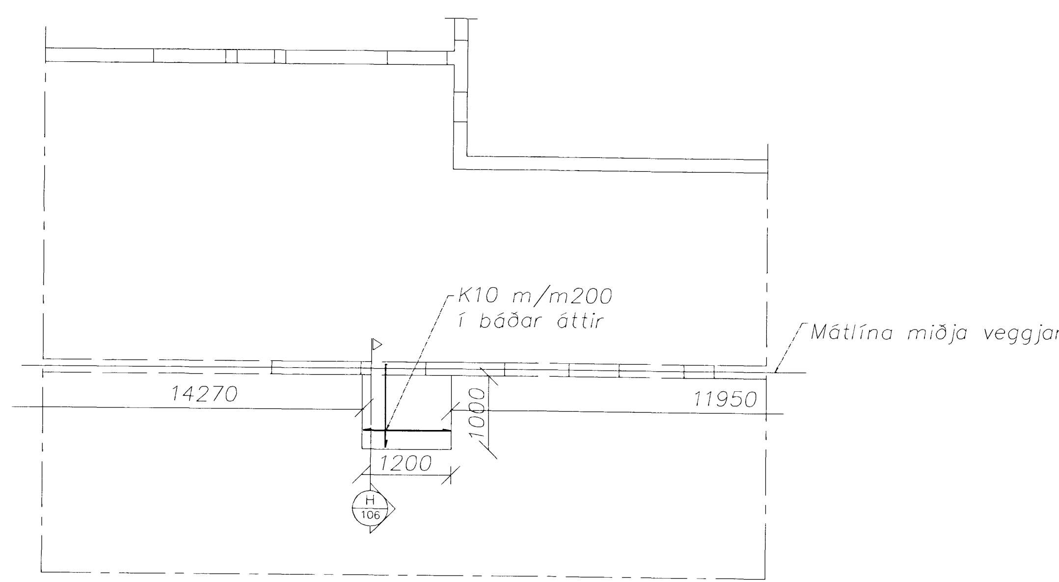
Grunnmynd milliþlata Mælikvarði 1:50
