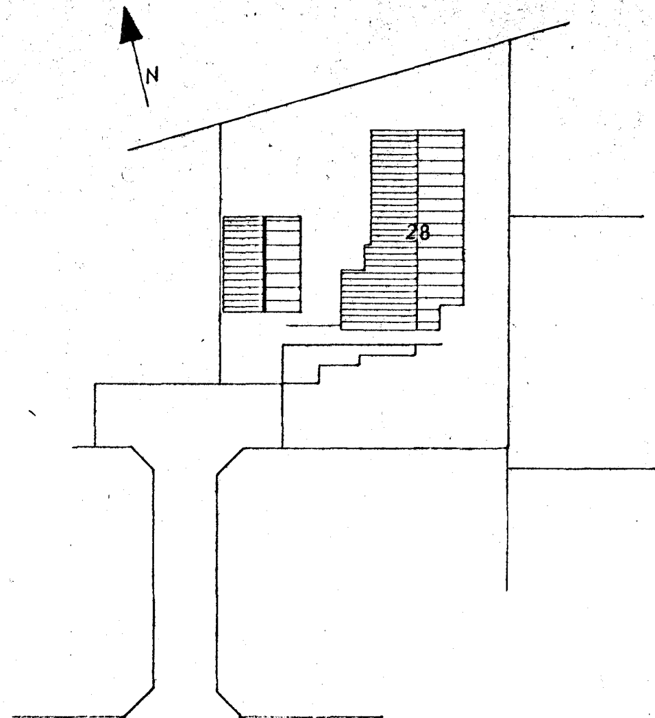
AFSTADA 1:500 NORÐURVANGUR
