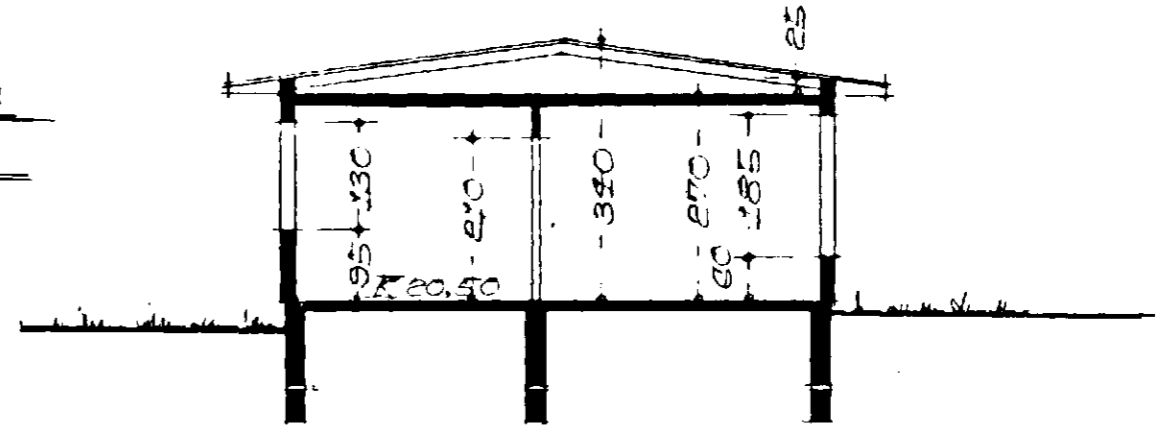
SNÍÐ A-A M=1:100
