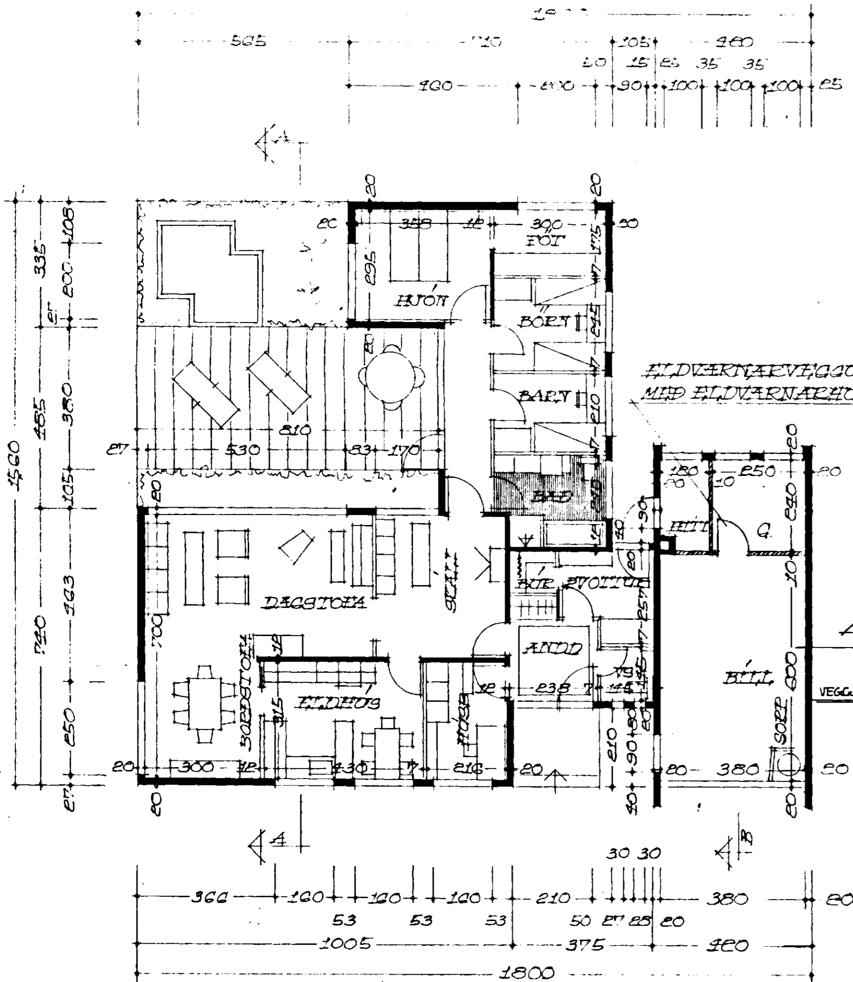
GRUNNMYND M=1:100
