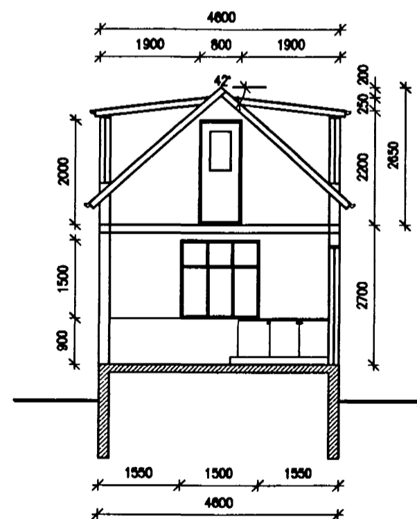
SNIÐ A-A
