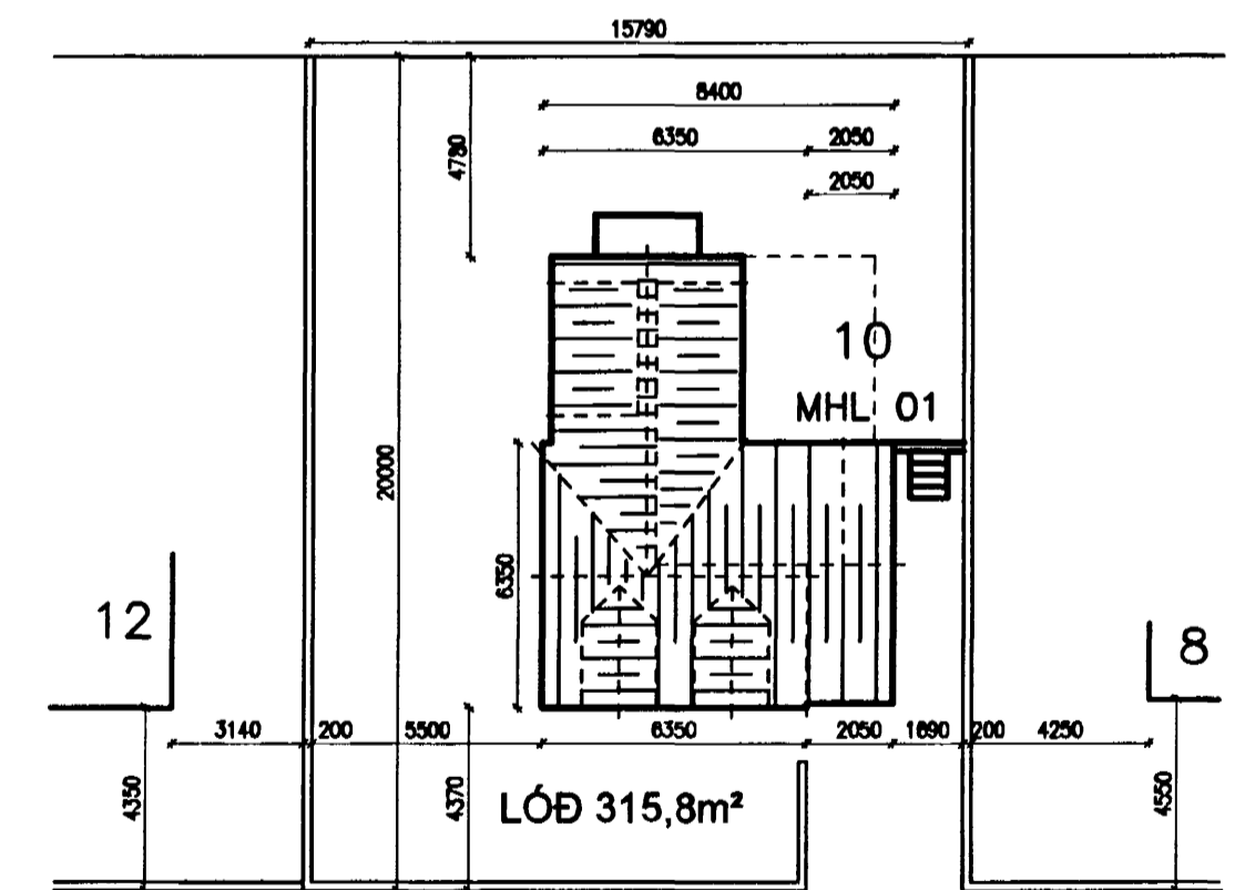
AFSTÖÐUMYND, 1:200
