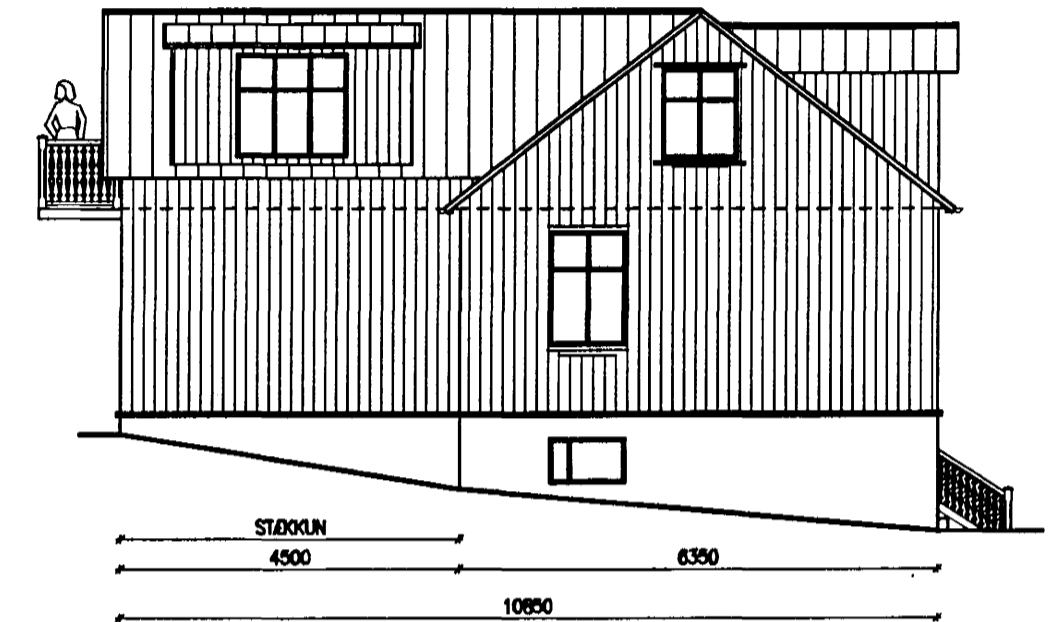
AUSTURGAFL
