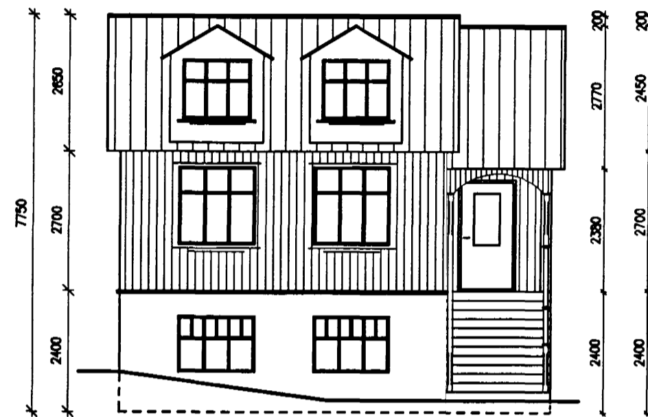
FRAMHLIÐ
