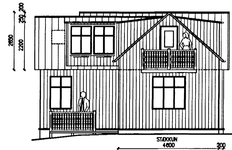
BAKHLIÐ
