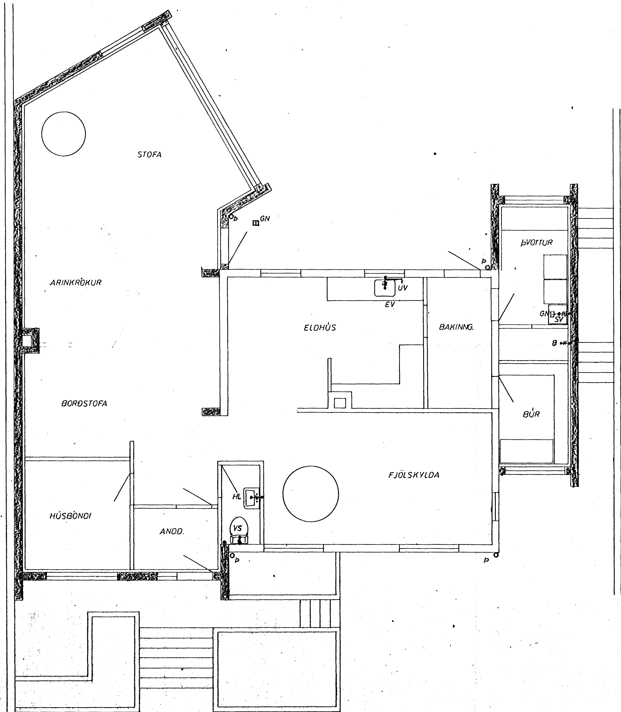
GRUNNMYND 1 HÆÐ 1:50
