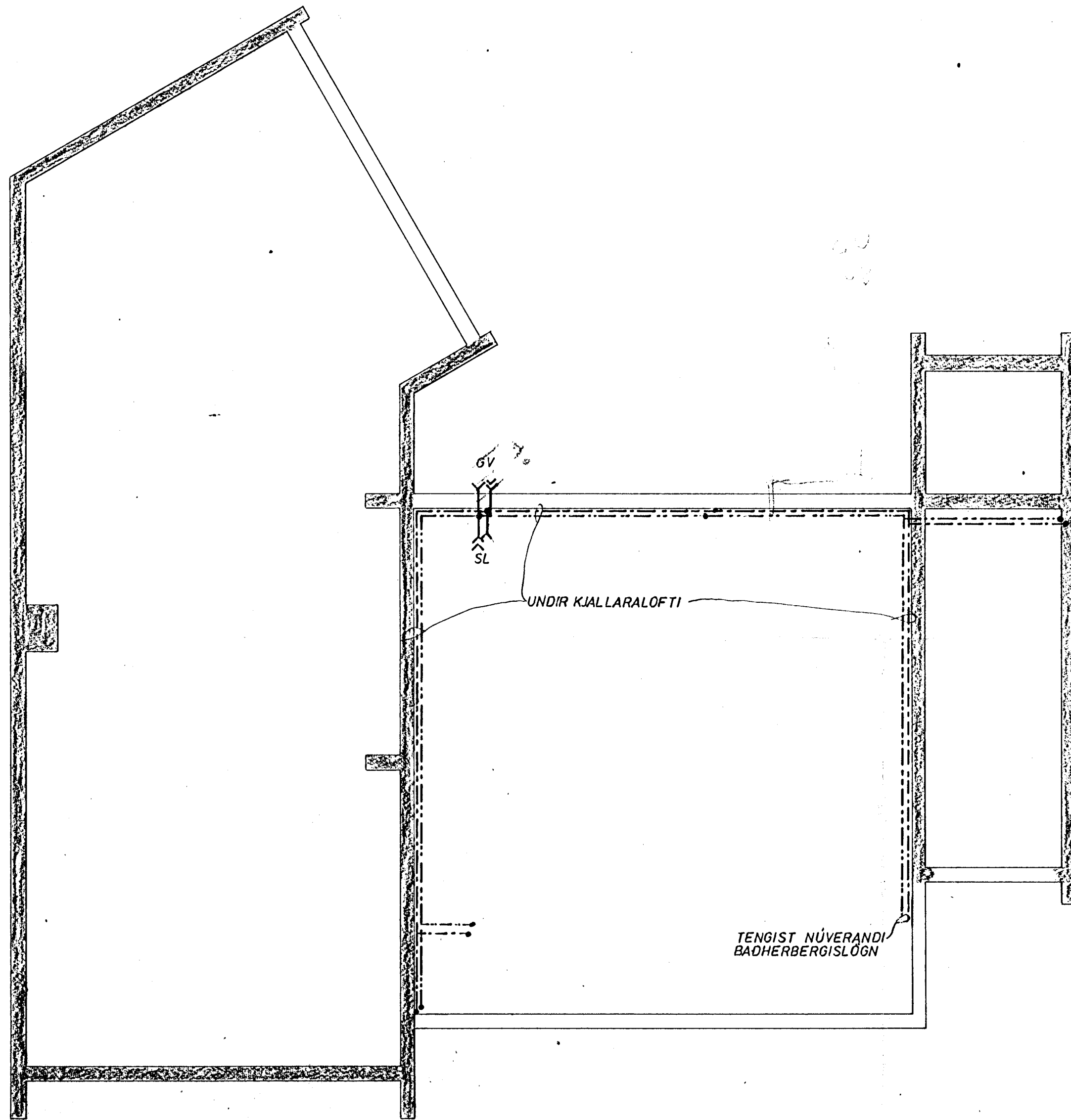
GRUNNMYND KJALLARA 1:50
