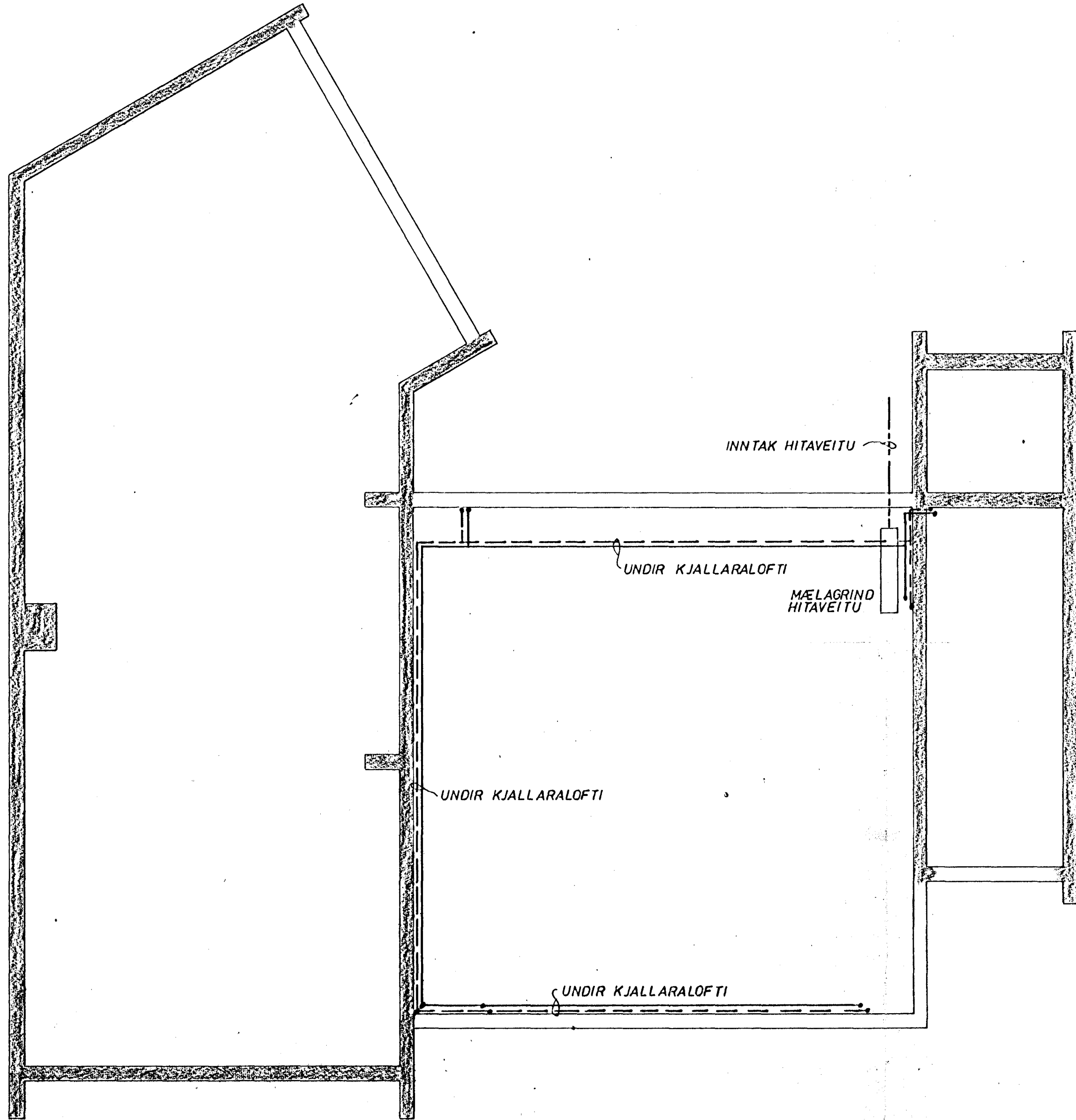
GRUNNMYND KJALLARA 1:50
