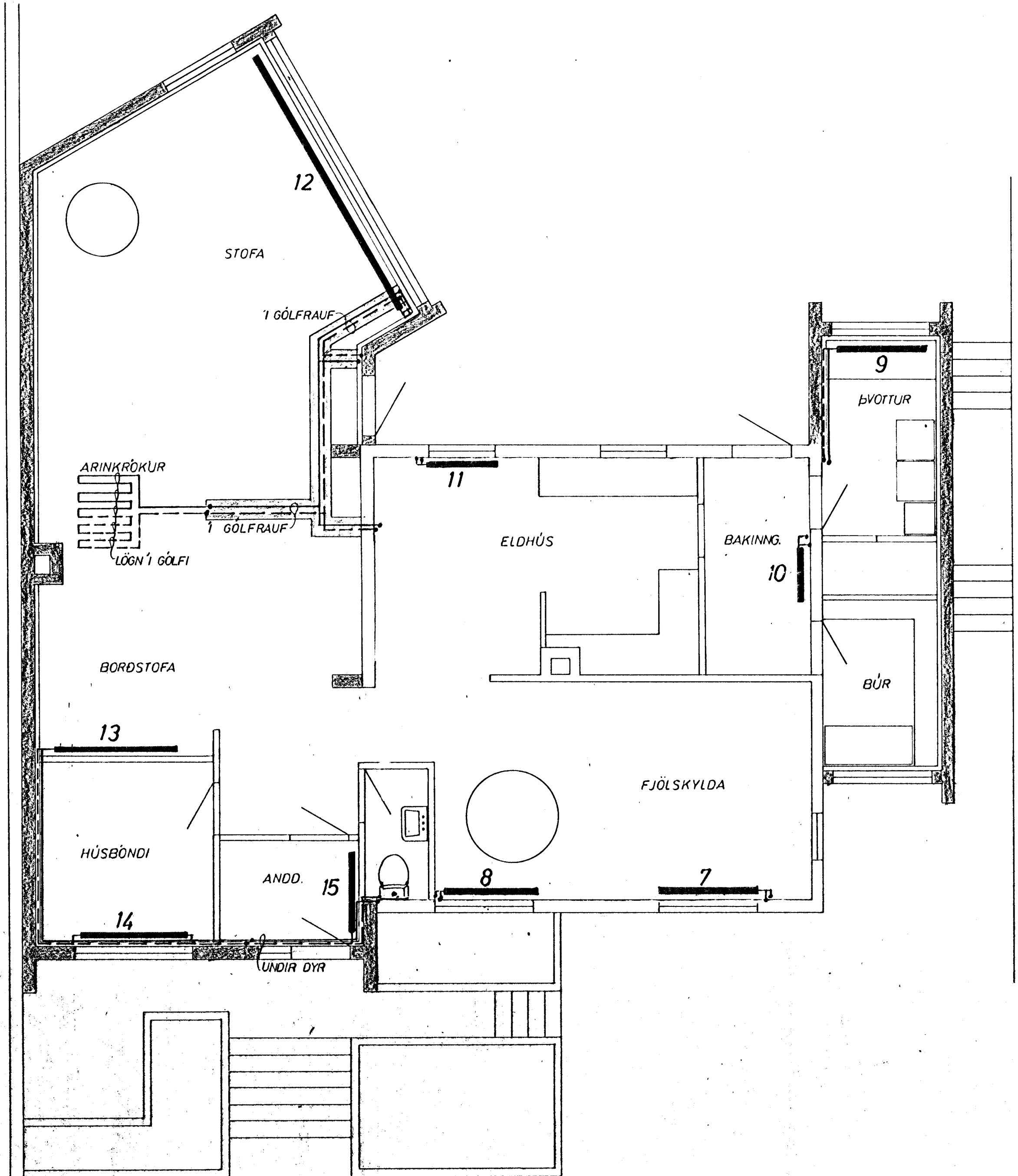
GRUNNMYND 1 HÆÐ 1:50
