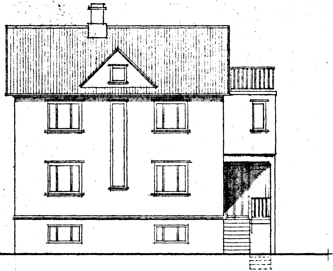
INNGANGSSMÍÐI FRÁ ÖLDUGÓTU
