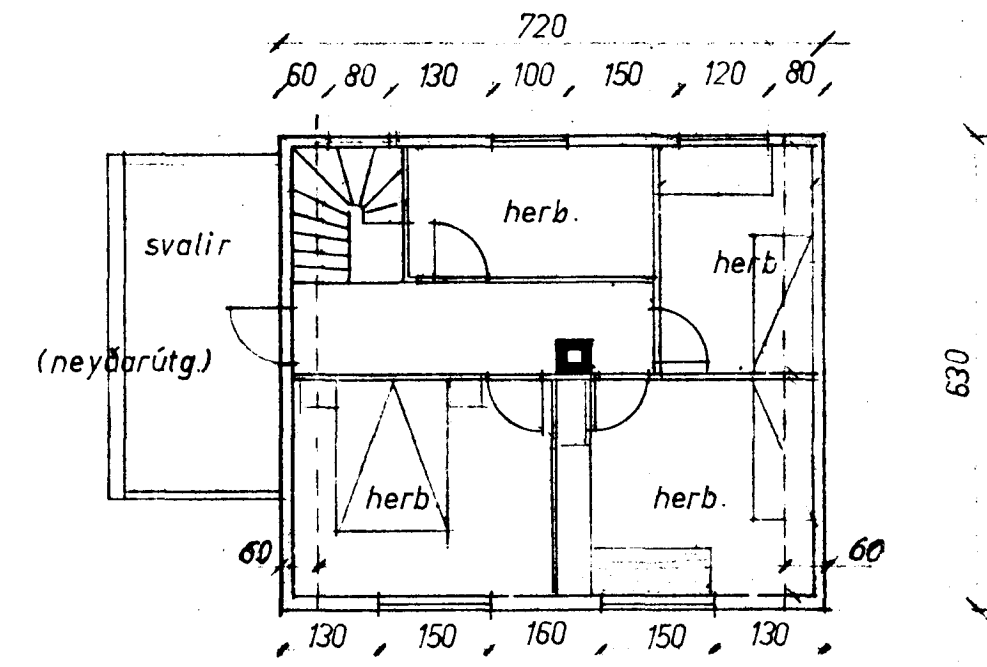
2. HÆÐ
