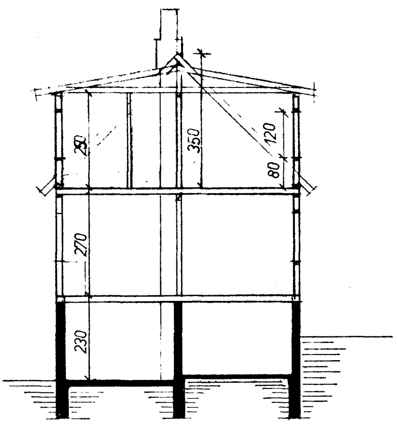
SNEIÐING B-B
