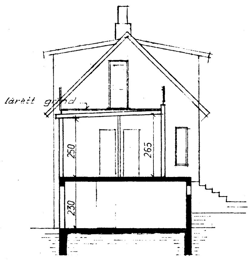
SNEIÐING A-A
