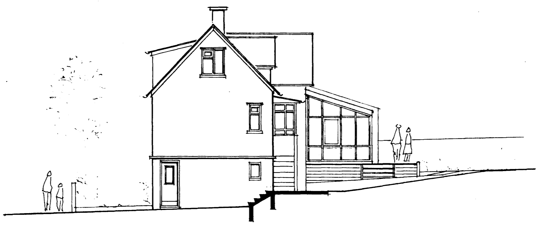
NORÐVESTUR M. 1:100
