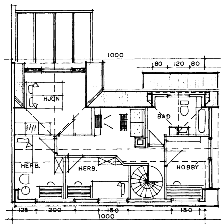
GRUNNMYND 2. HÆÐ M. 1:100
