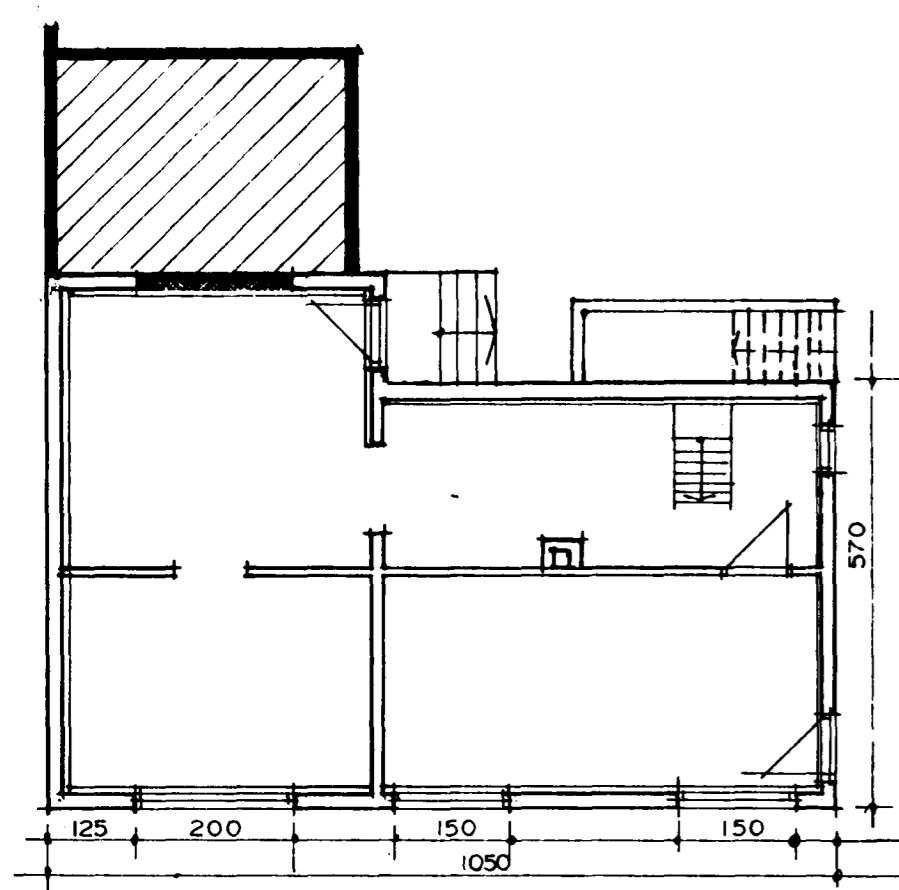
GRUNNMYND KJALLARI M. 1:100
