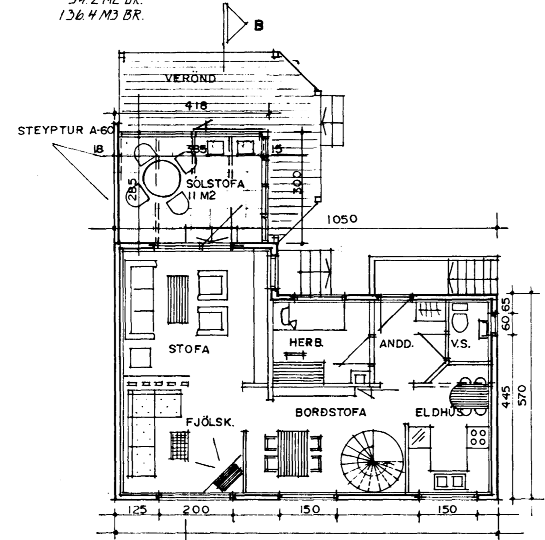
GRUNNMYND I. HÆÐ M. 1:100
