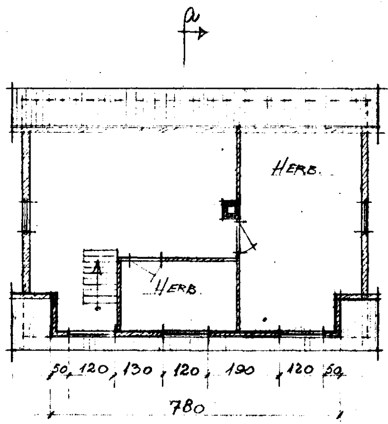
GRUNNMYND-RIS KVARDI 1:8100
