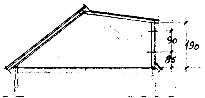
SNID a-a
