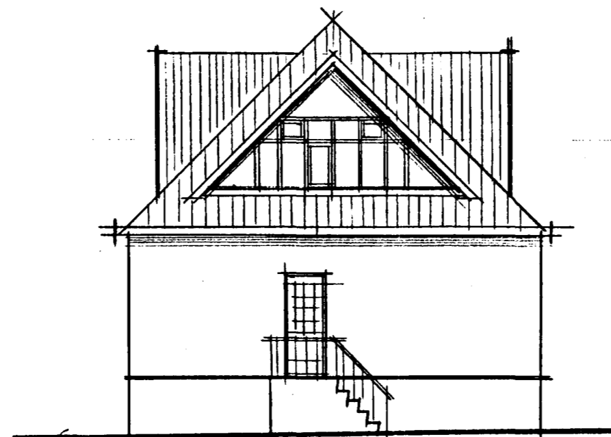
UTLIT NORDUR M=1:100
