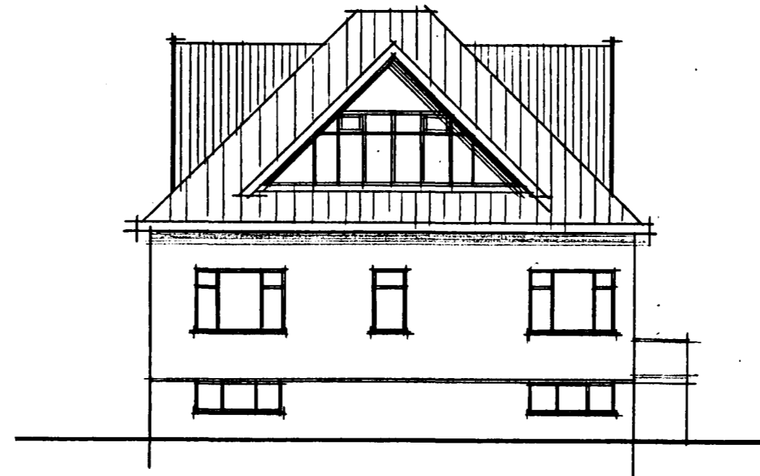
UTLIT AUSTUR M=1:100
