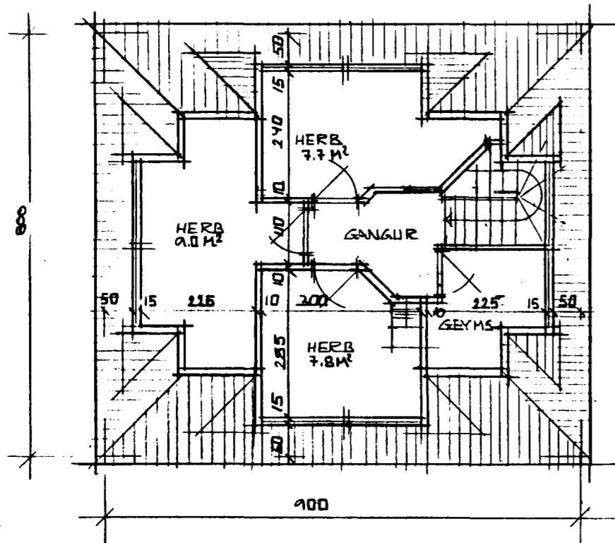
GRUNNMYND 2. HEDAR M=1:100
