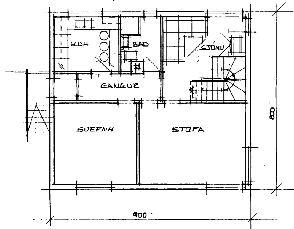
GEUNNMYND 1. HEDAR M=1:100
