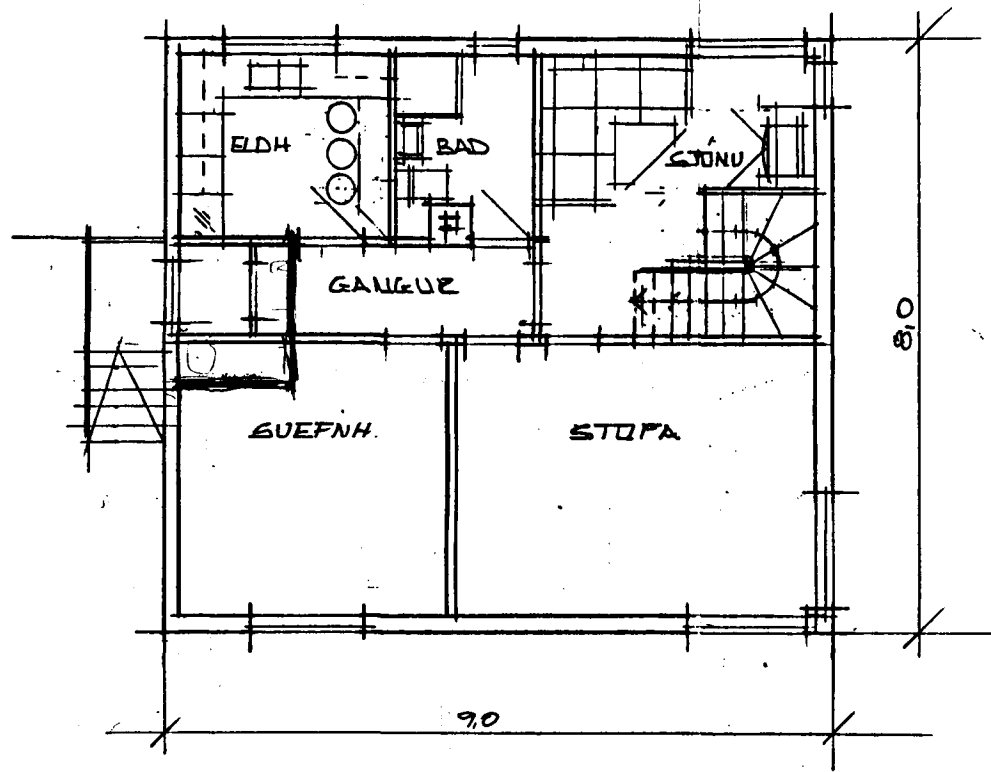
GEUNNMYND 1. HÆÐAR M=1:100
