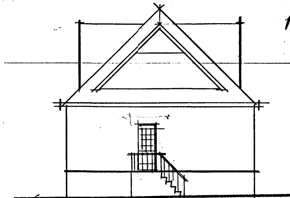
ÚTLIT NORDUR M=1:100
