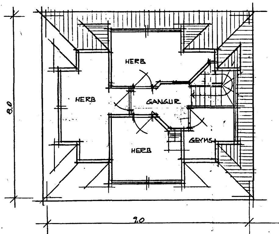
GEUNNMYND 2. HÆÐAR M=1:100
