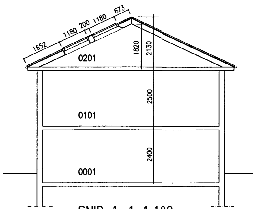
SNID 1-1 1:100
