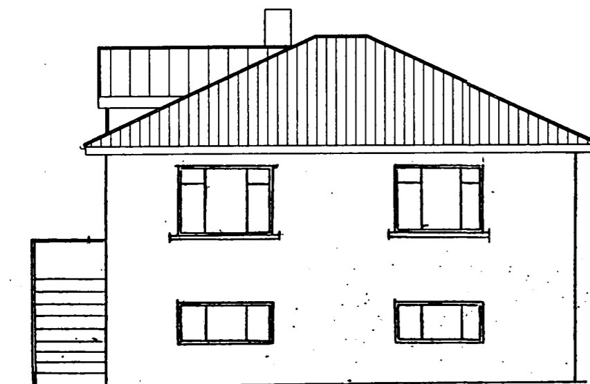
SUÐVESTUR
