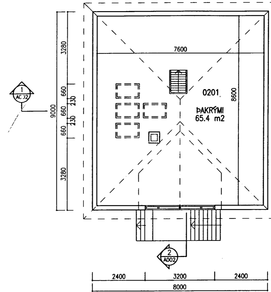
GRUNNMYND ÞAKRÝMI 1:100
