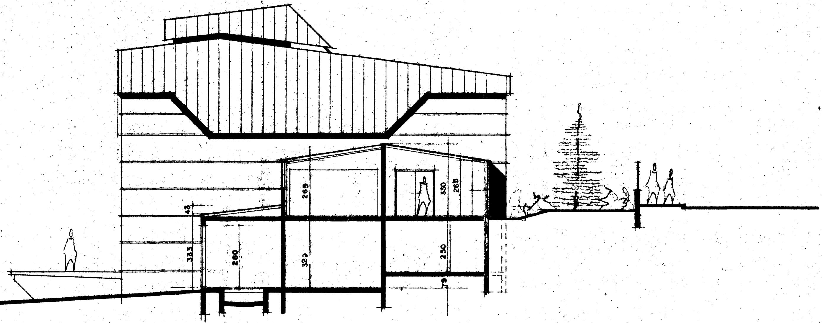
útlit norð-vestur / snið D-D m=1:100
