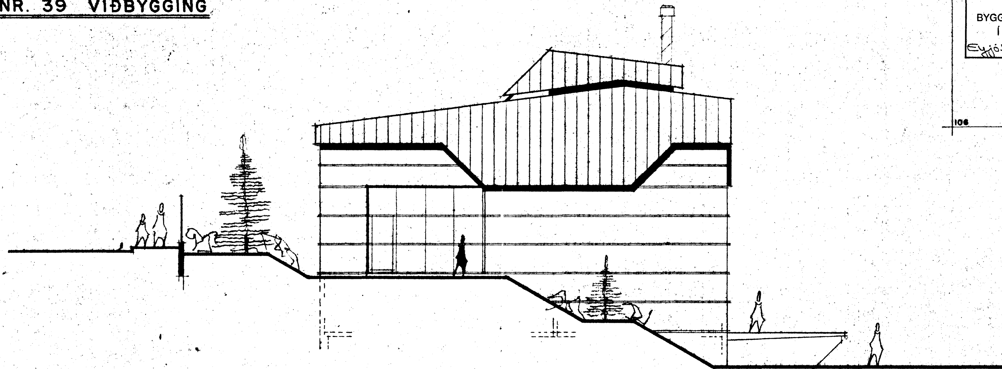
útlit suð-austur m=1:100
