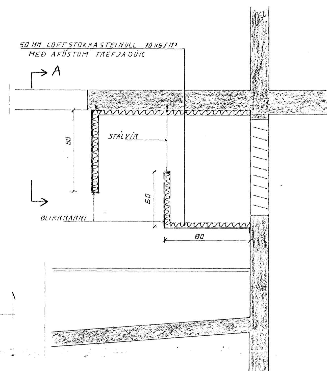
SNID 1 1:20. HLJÓÐGILDRÁ VIÐ LOFTINNTAK
