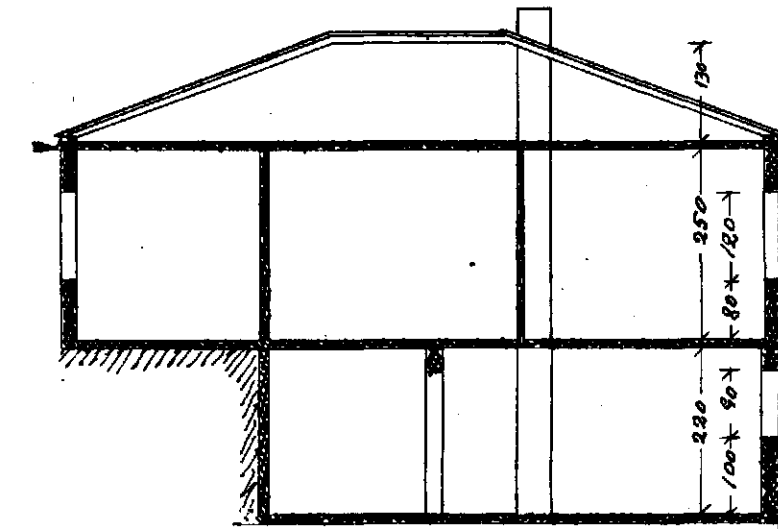
Skurður a-a
