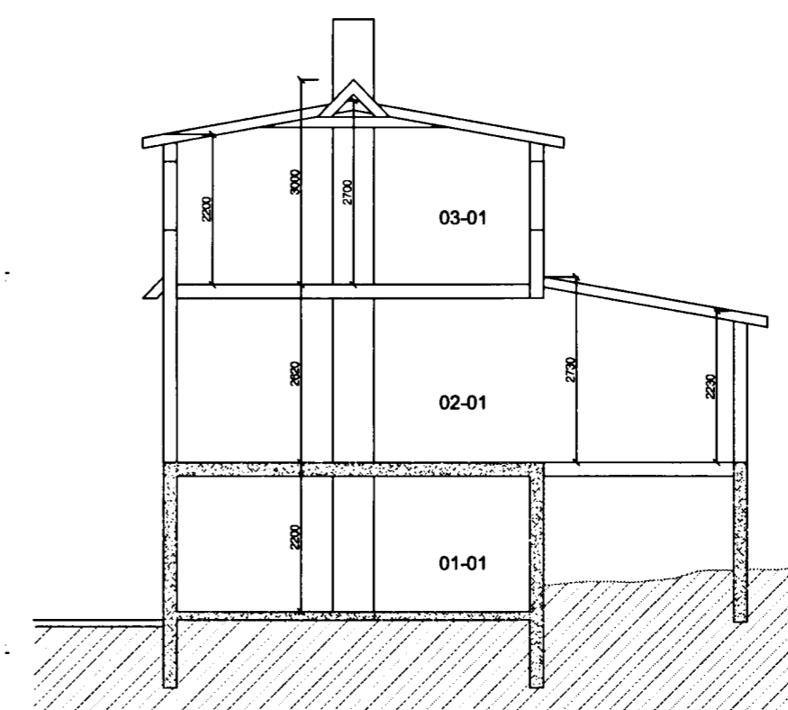
SNEIÐING A-A
