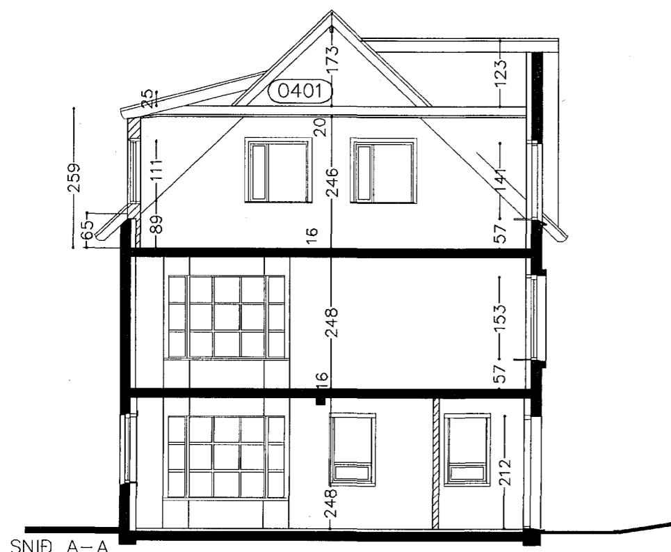
SNID A-A
