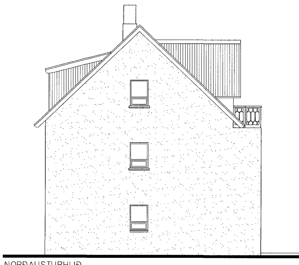
NORÐAUSTURHLIÐ
