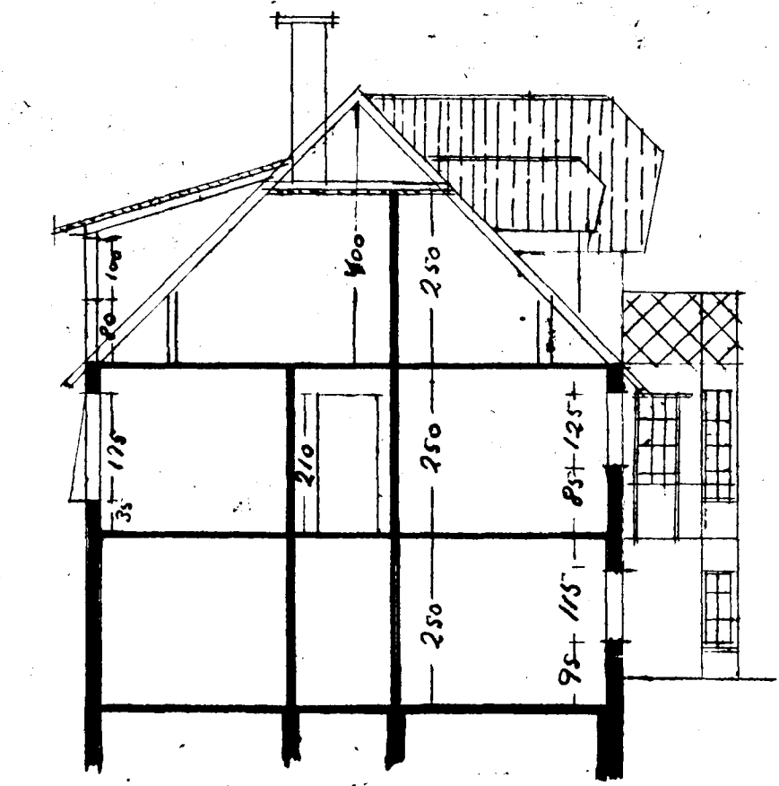
Skurður A-A.
