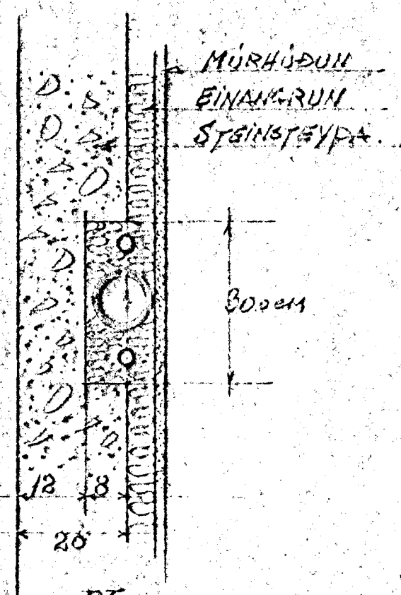
VEGGRAND FIRIR VATNS-OG SKOLPLAGNIR I UTVEGG KVARDI 1:10
