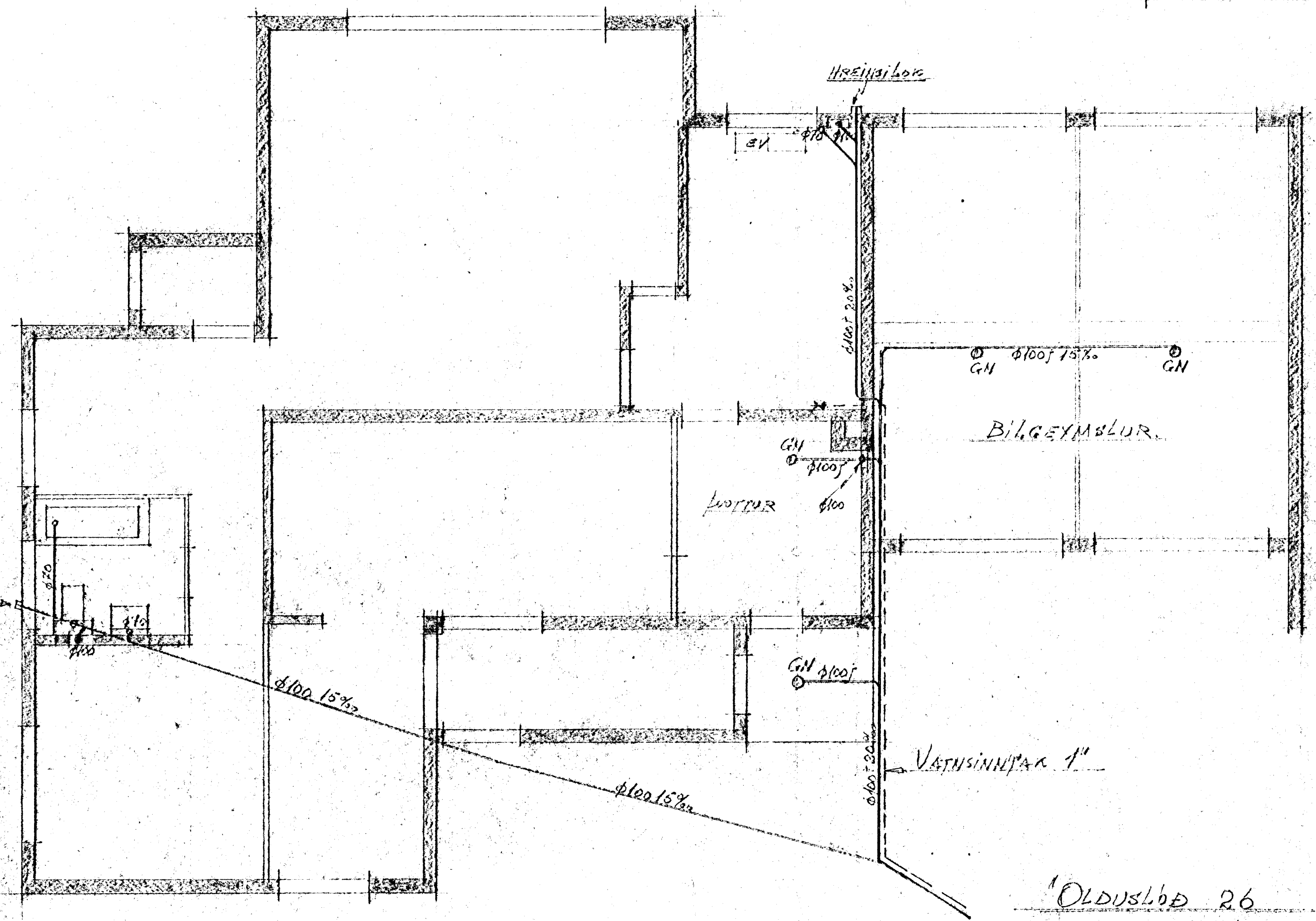
GRUNNMÝND, KVARDI 1:50
