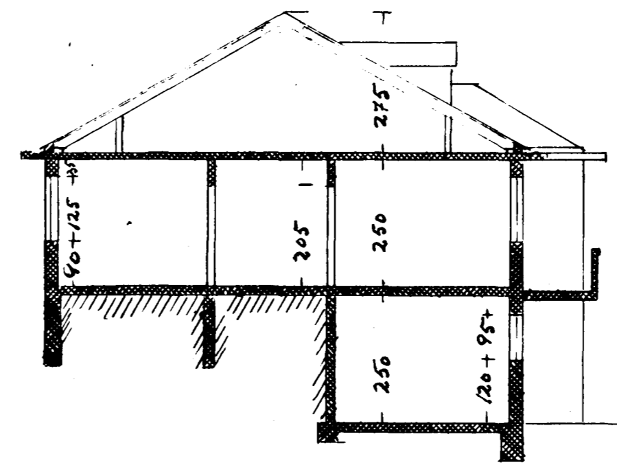
Sneiðing A.A.
