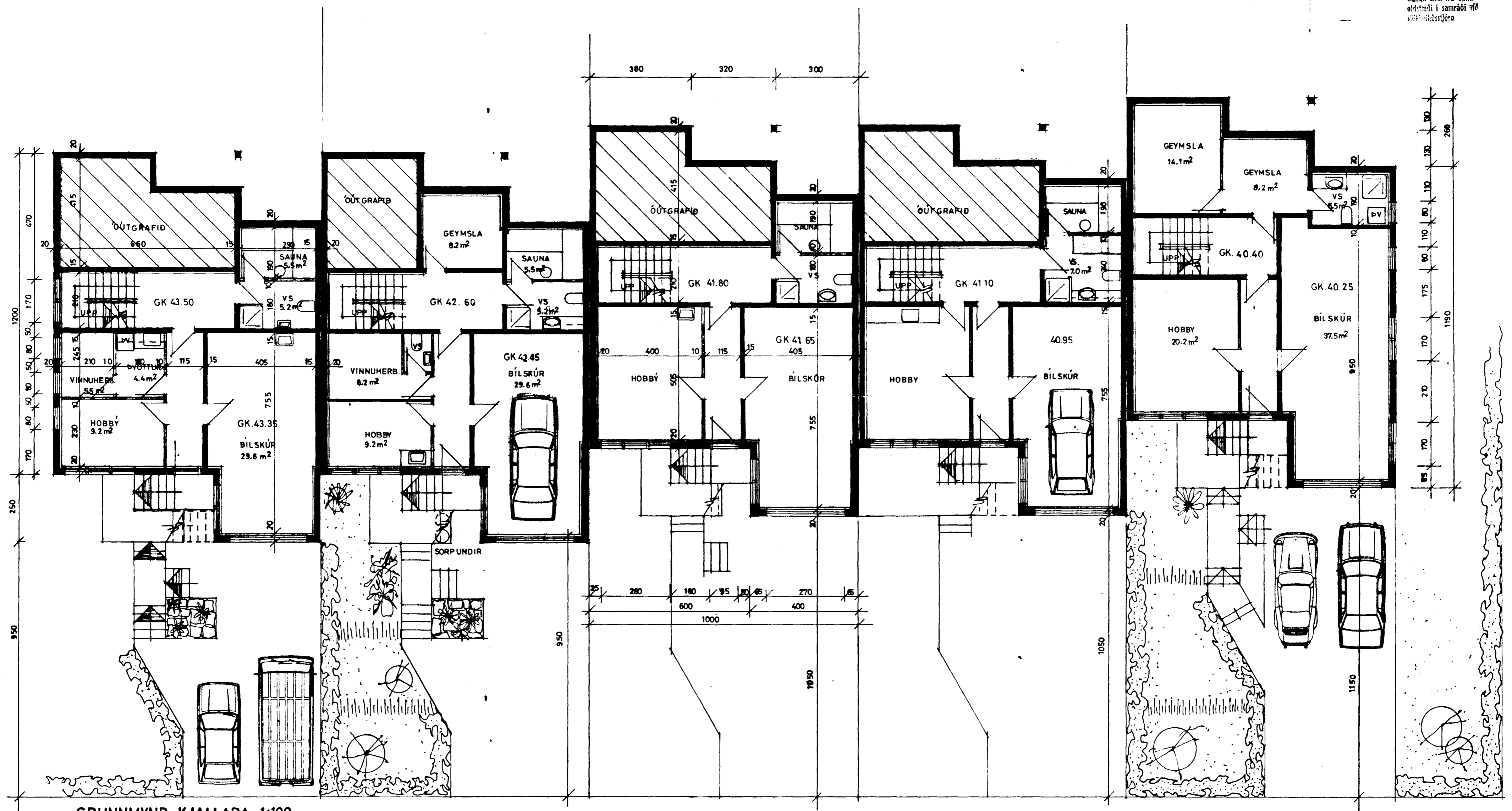
GRUNNMYND KJALLARA 1:100
