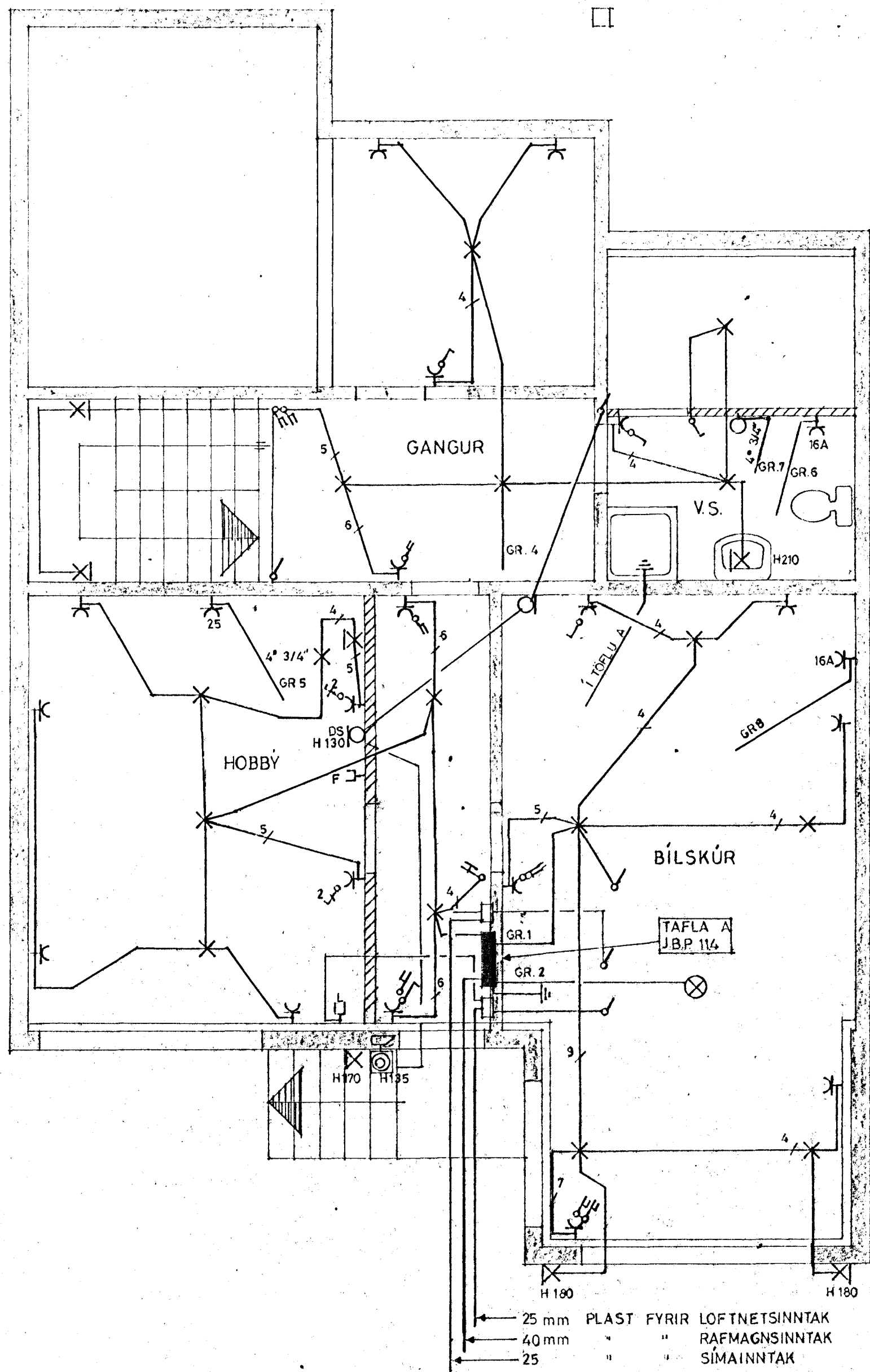
GRUNNMYND KJALLARA 1:50
