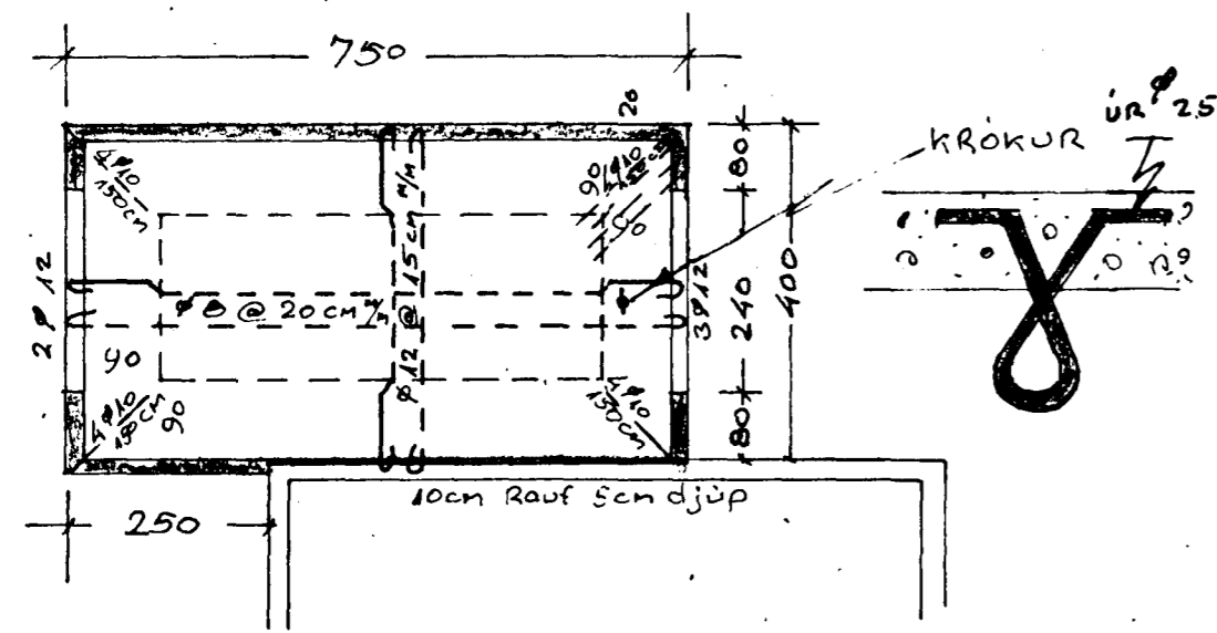
BILGEYMSLA
