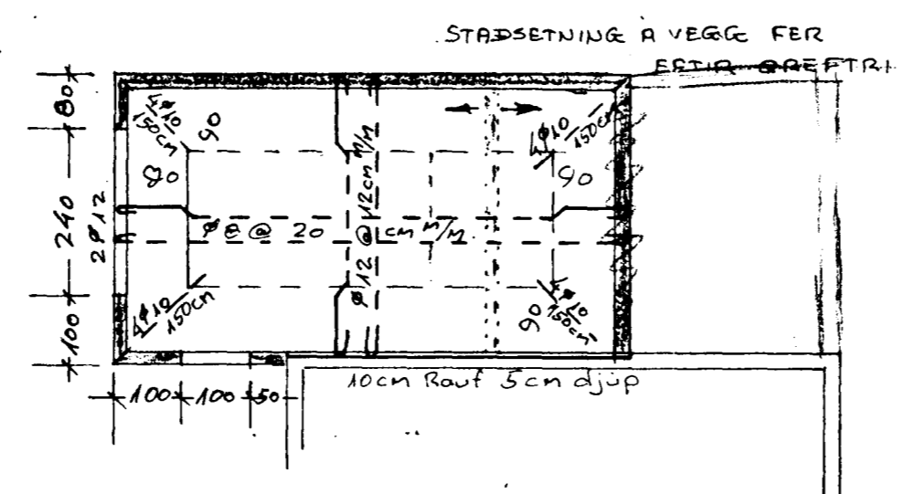
KJALLARI
