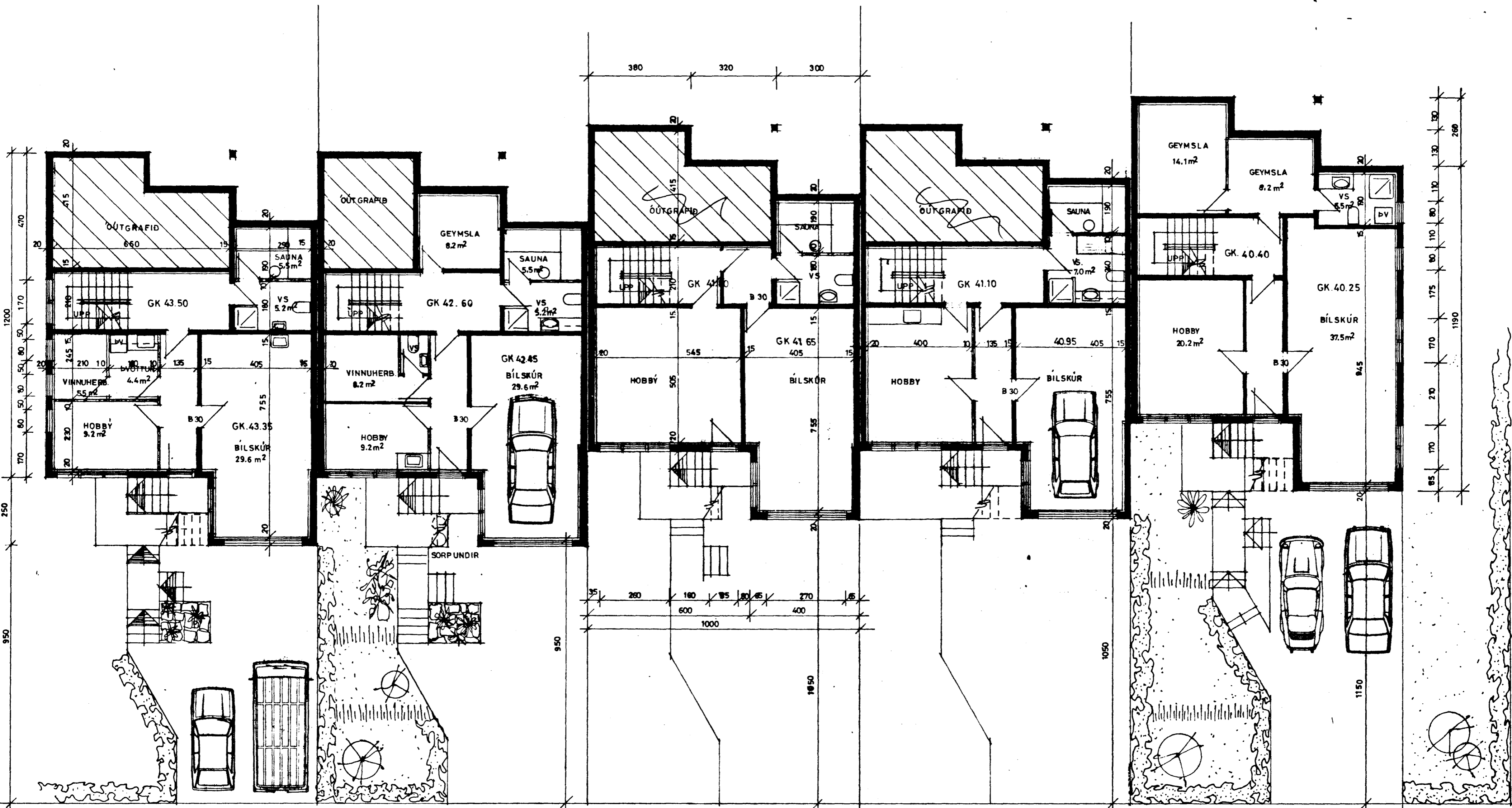
GRUNNMYND KJALLARA 1:100
