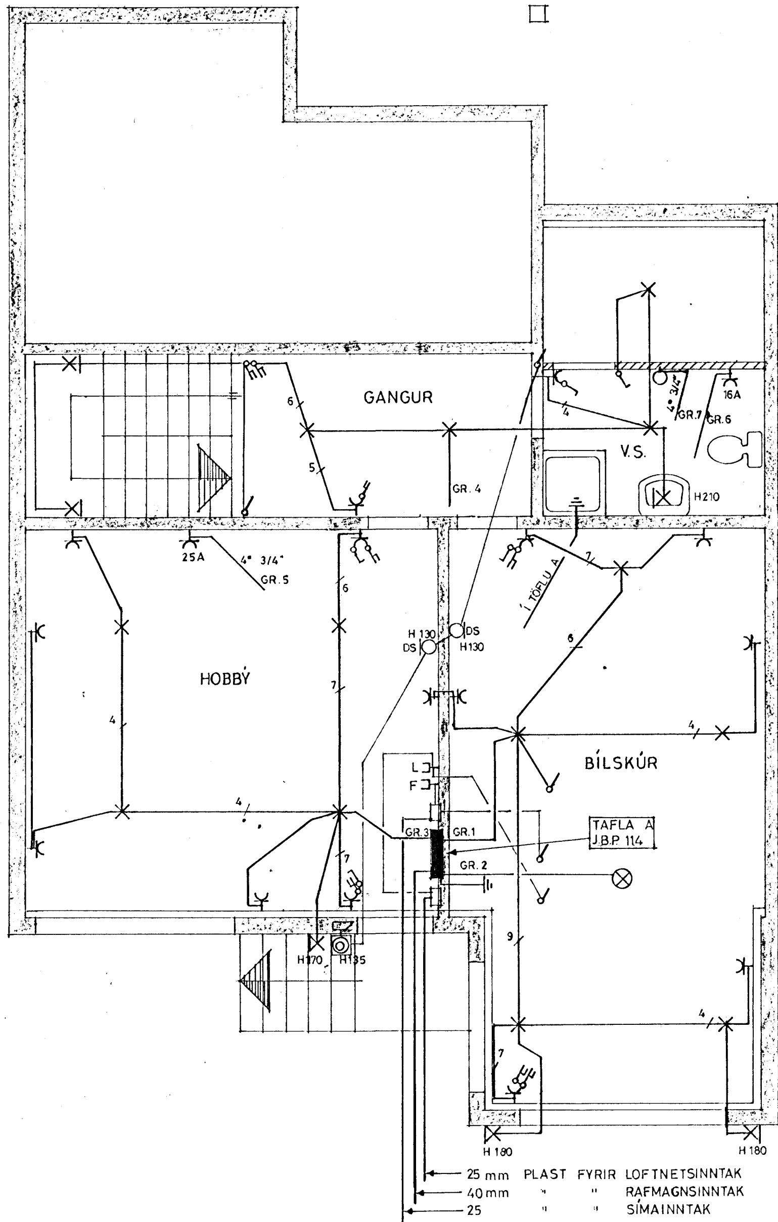
GRUNNMYND KJALLARA 1:50
