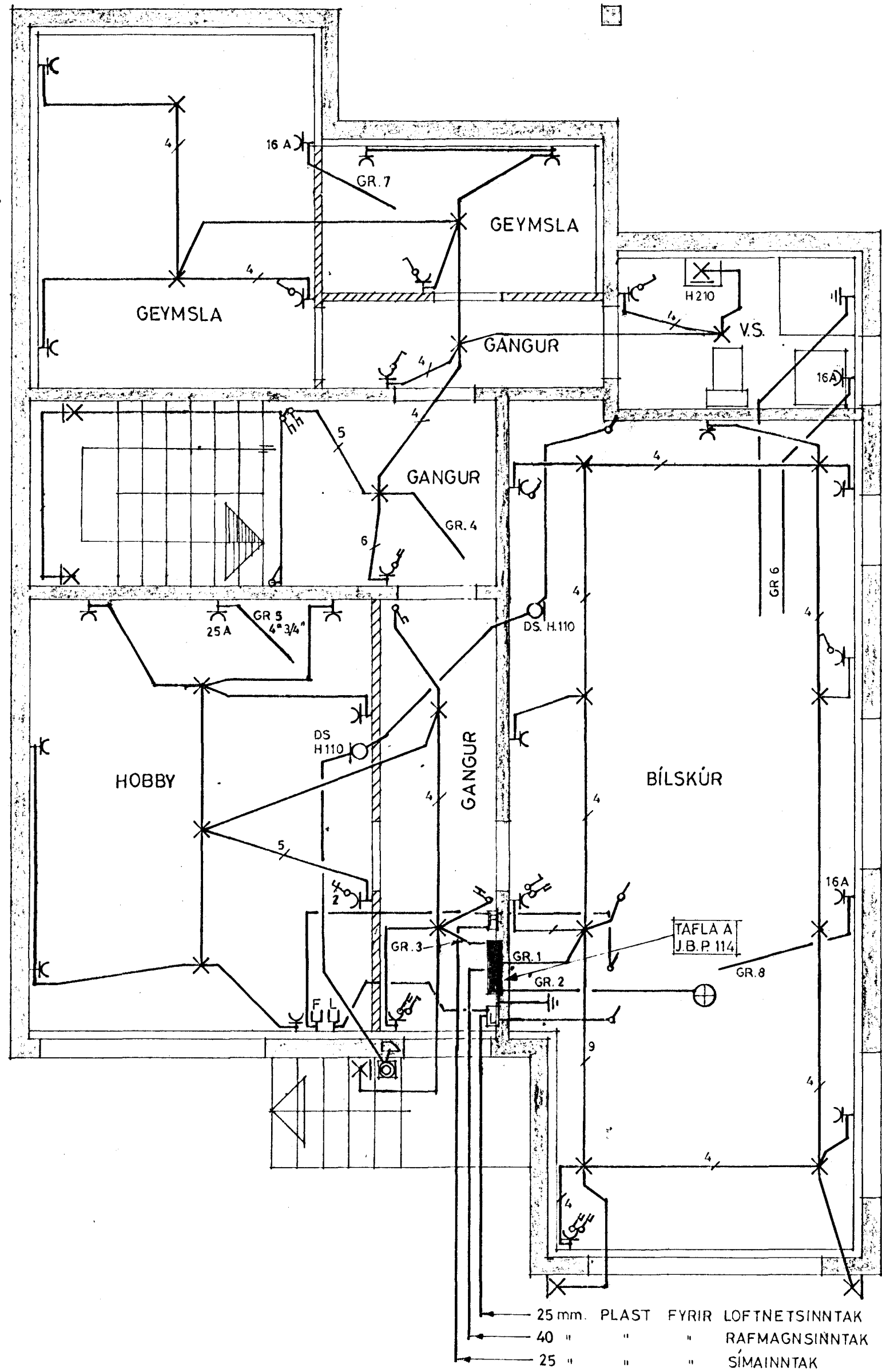
GRUNNMYND KJALLARA 1:50
