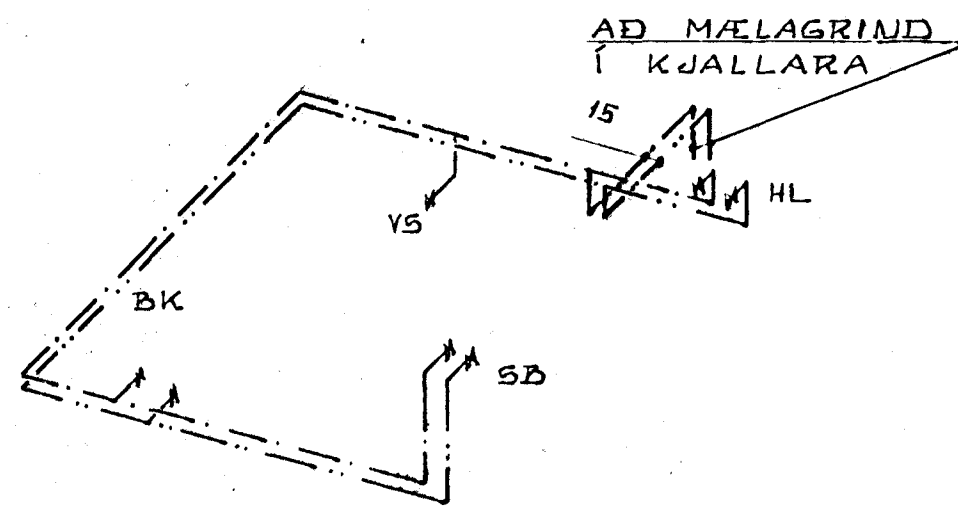
RÚMMYND VATNSLAGNA 1:50
