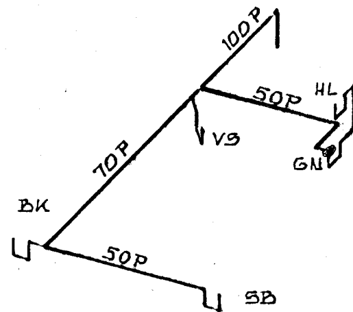
RÚMMYND FRÁRENNISLAGNA 1:50
