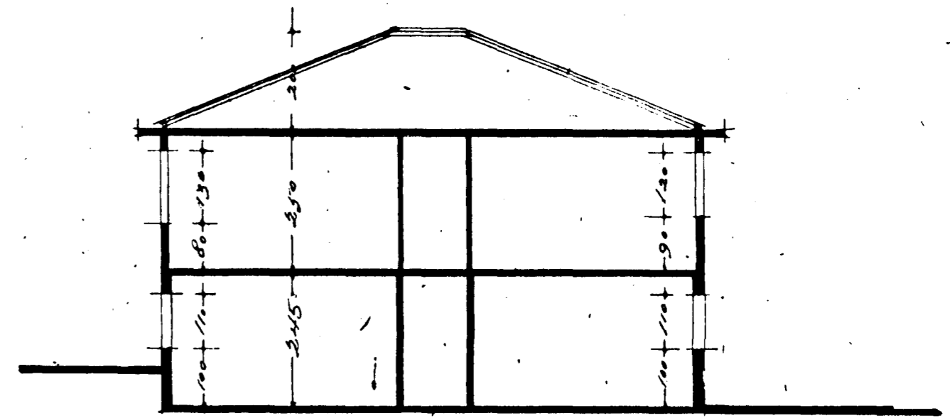
SNÍÐ A-B
