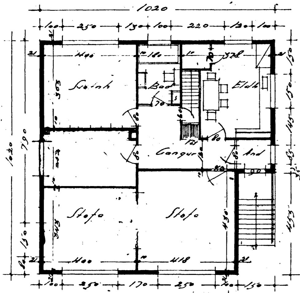
GRUNNUMYND 2. HÆÐAR
