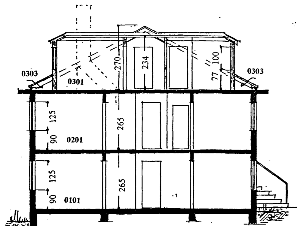
Snið: A-A
