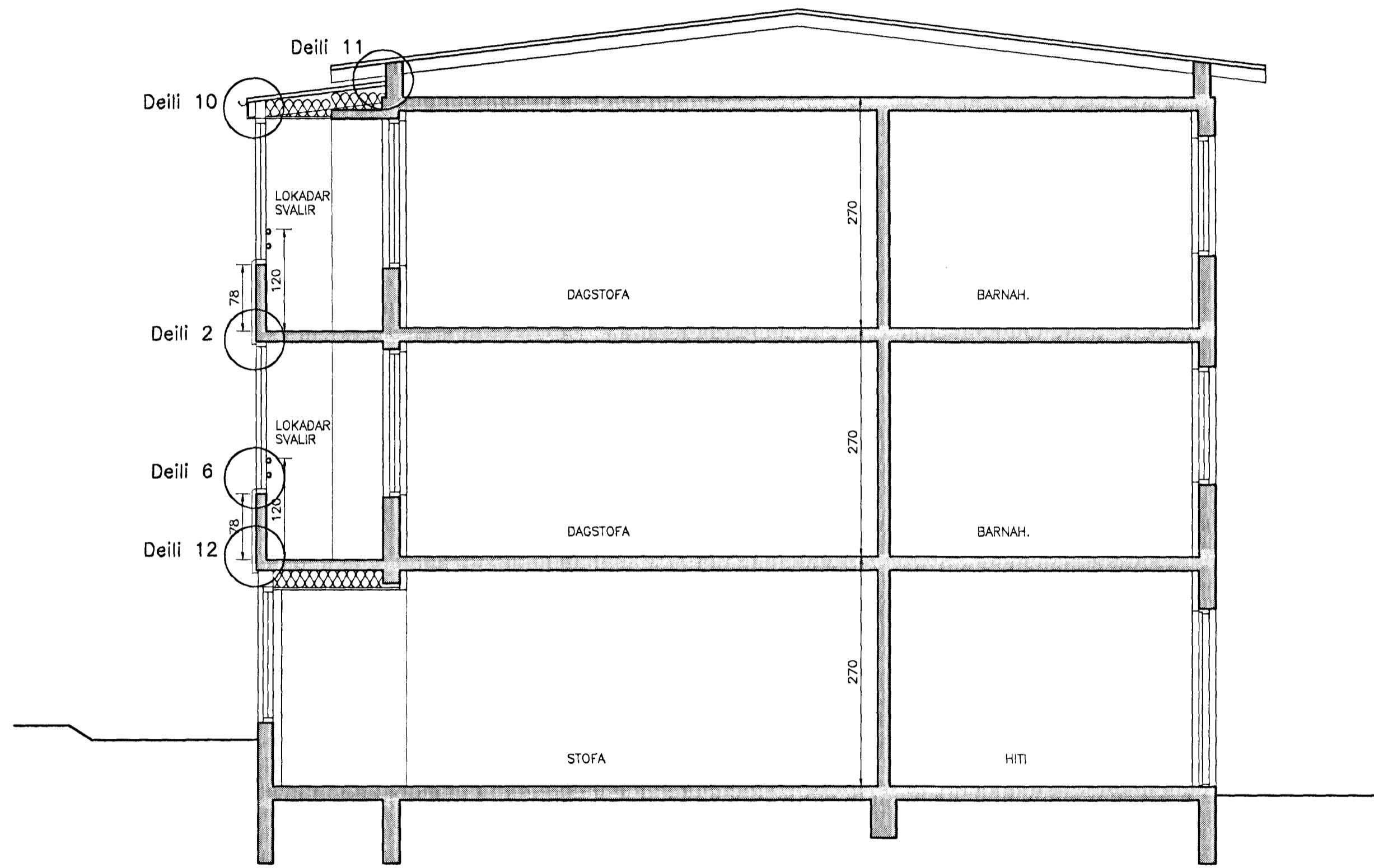
SNÍÐ A-A MKV. 1:50
