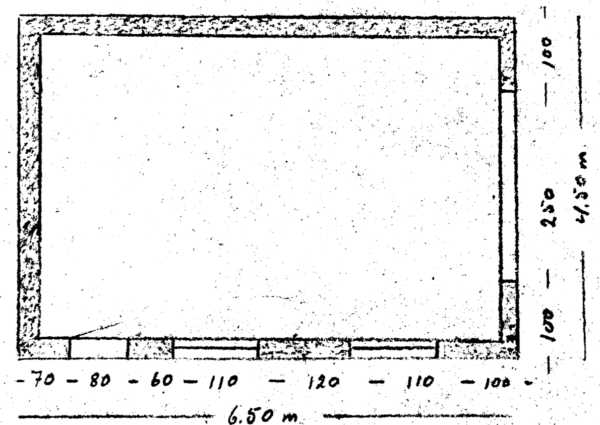
Grunnmynd.
