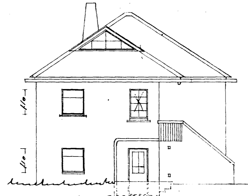
Norður.
