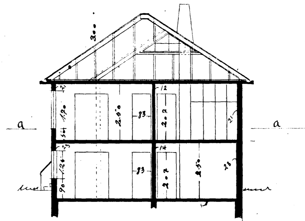
Þverskurður.
