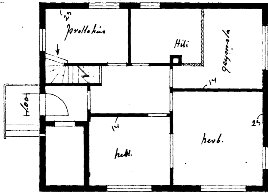
kjallari
