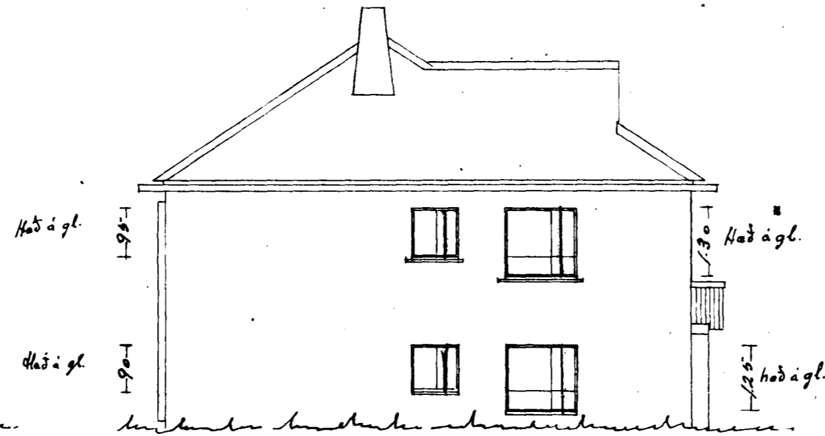
Austur.
