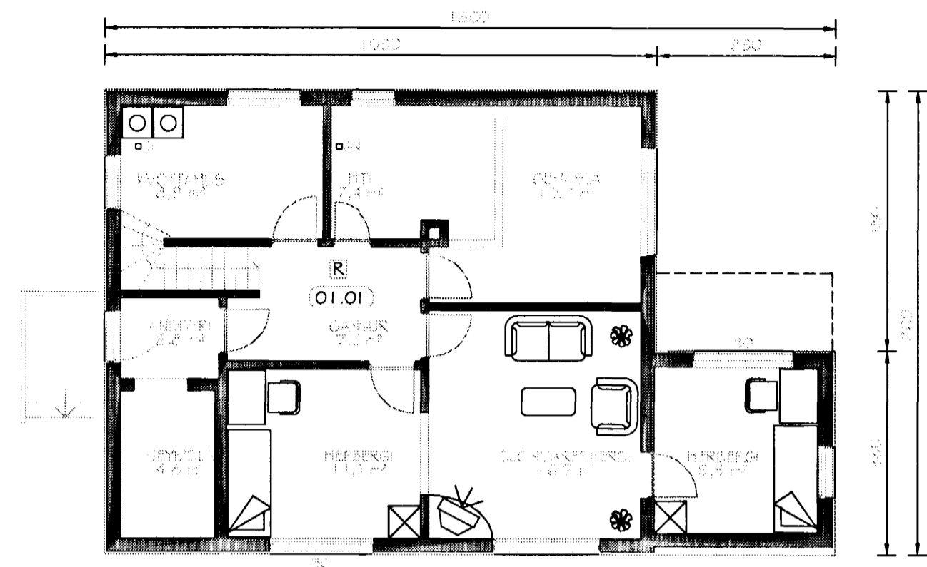
GRUNNMYND NEÐRI HÆÐAR
