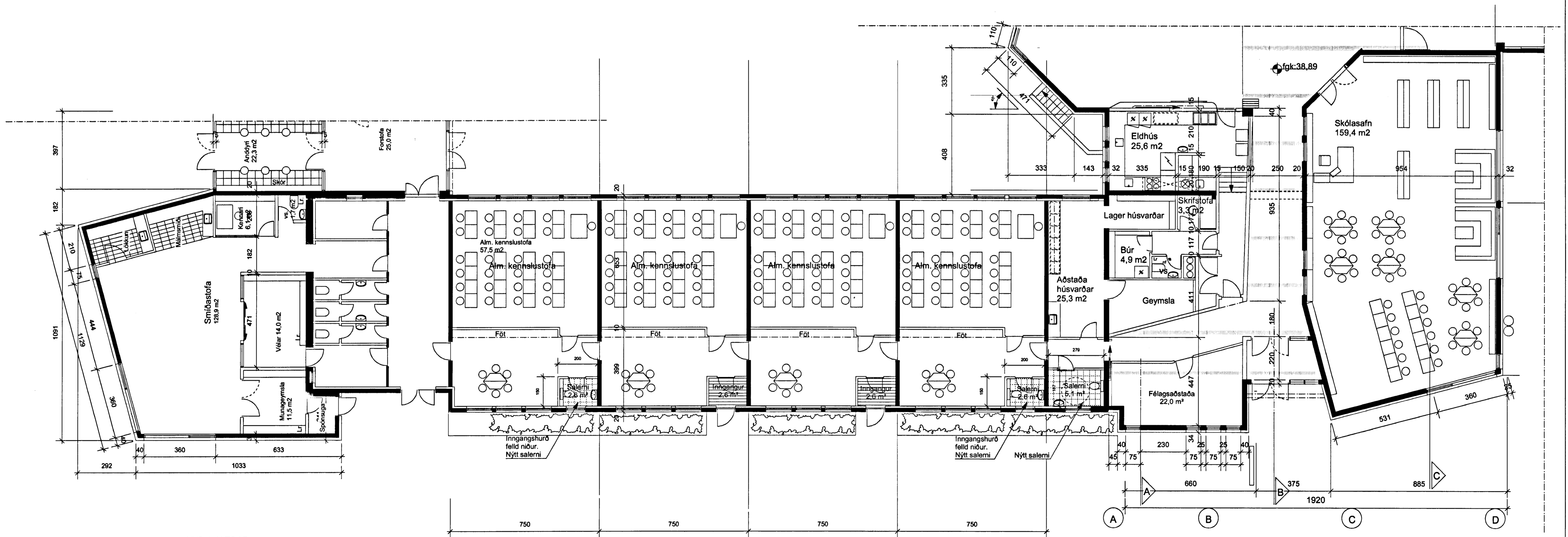
GRUNNMYND 1. HÆÐAR
