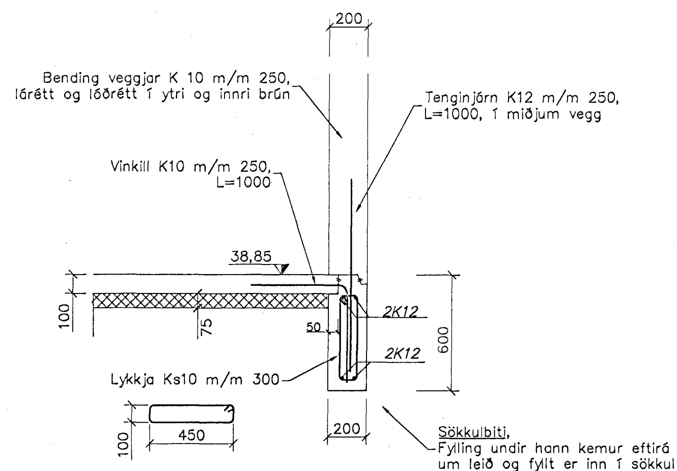
Snið A, 1:20
