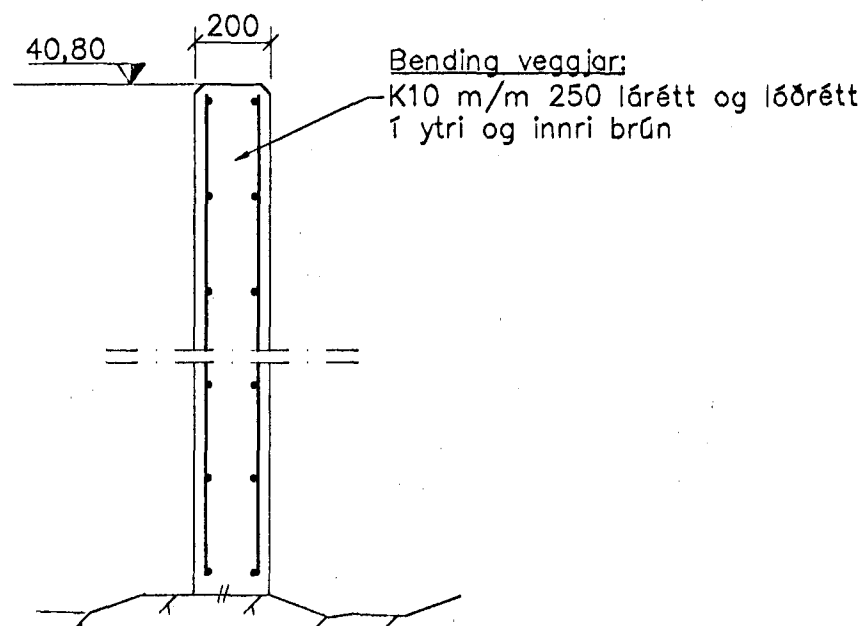
Snið J, 1:20
