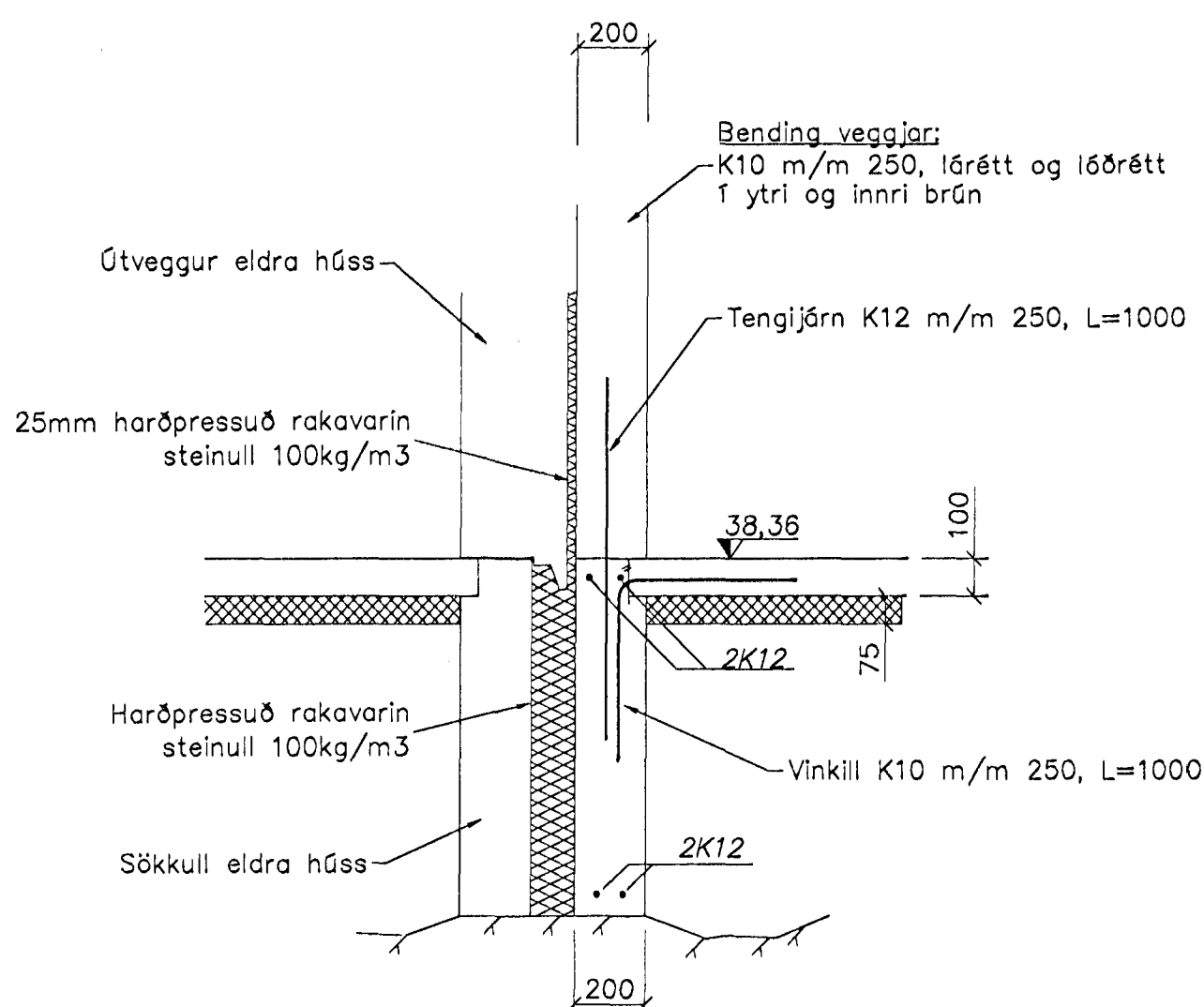
Snið F, 1:20
