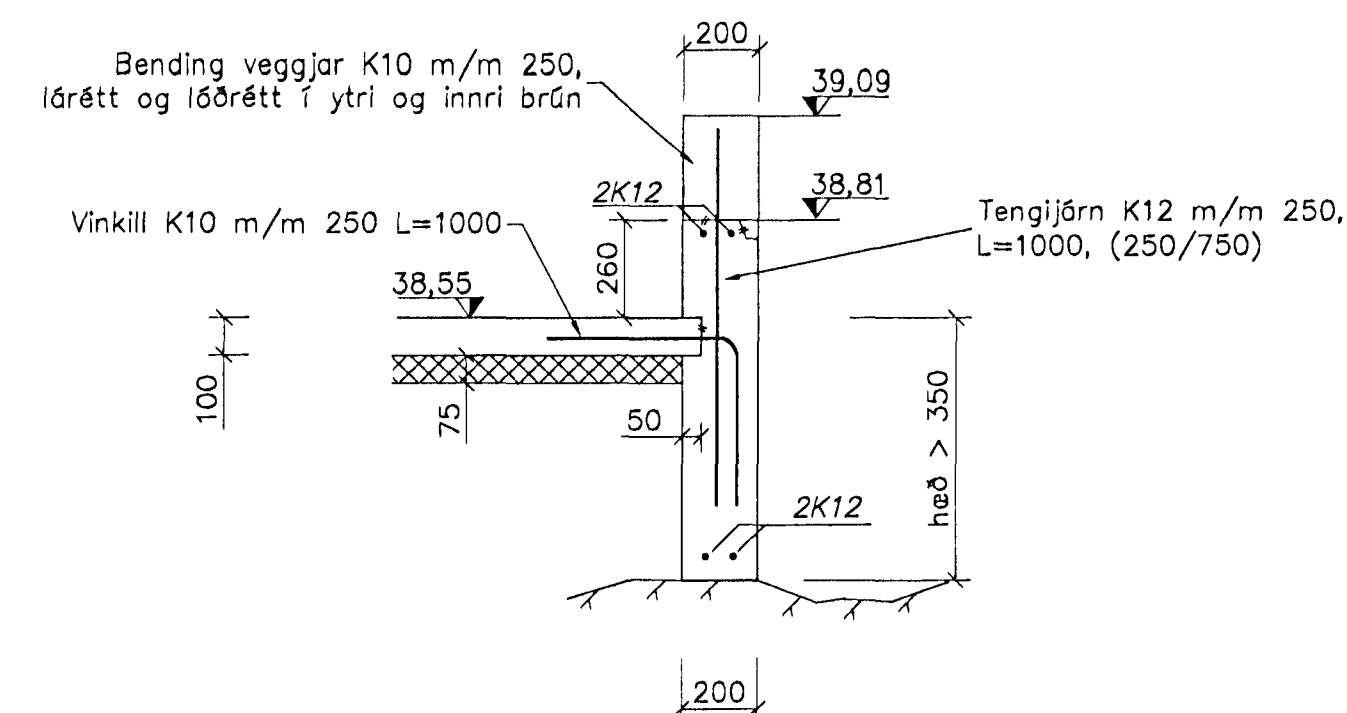
Snið D, 1:20
