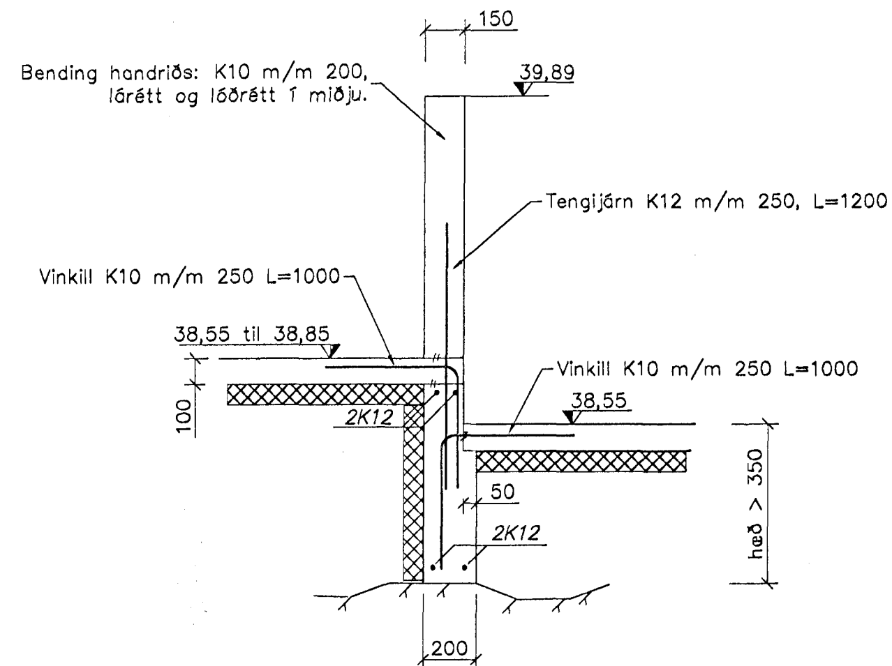
Snið I, 1:20
