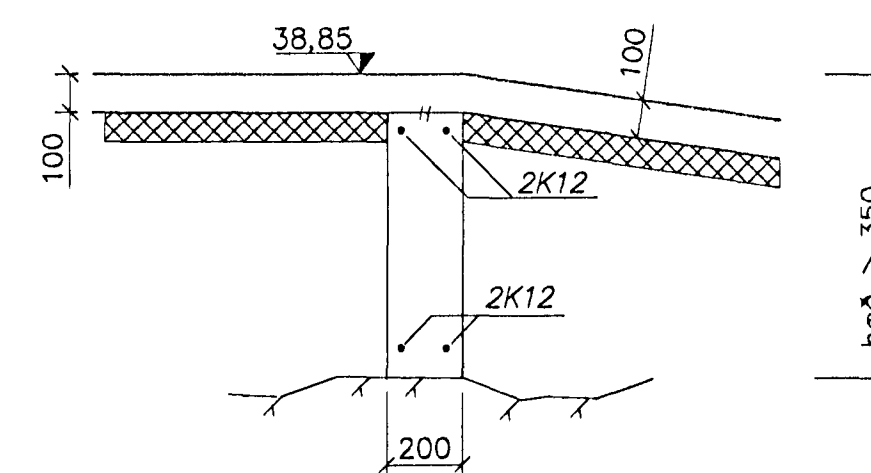
Snið H, 1:20
