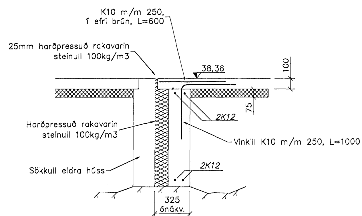
Snið G, 1:20
