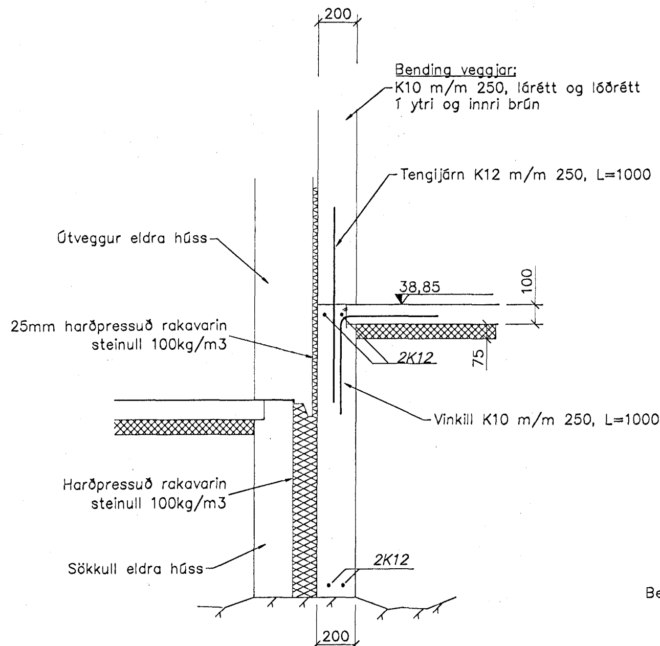
Snið E, 1:20
