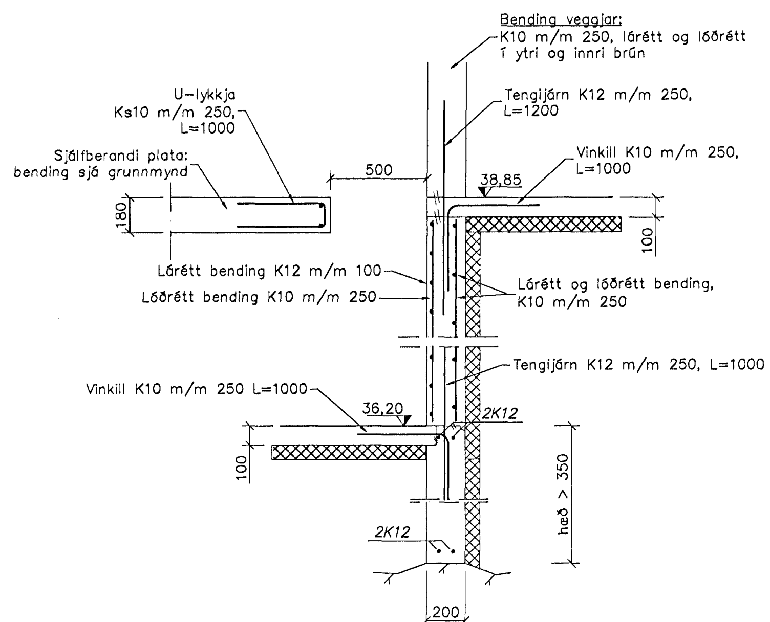
Snið K, 1:20
