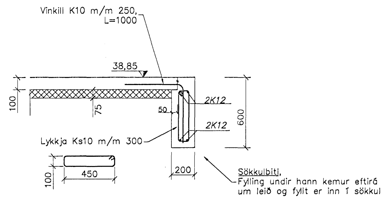
Snið B, 1:20
