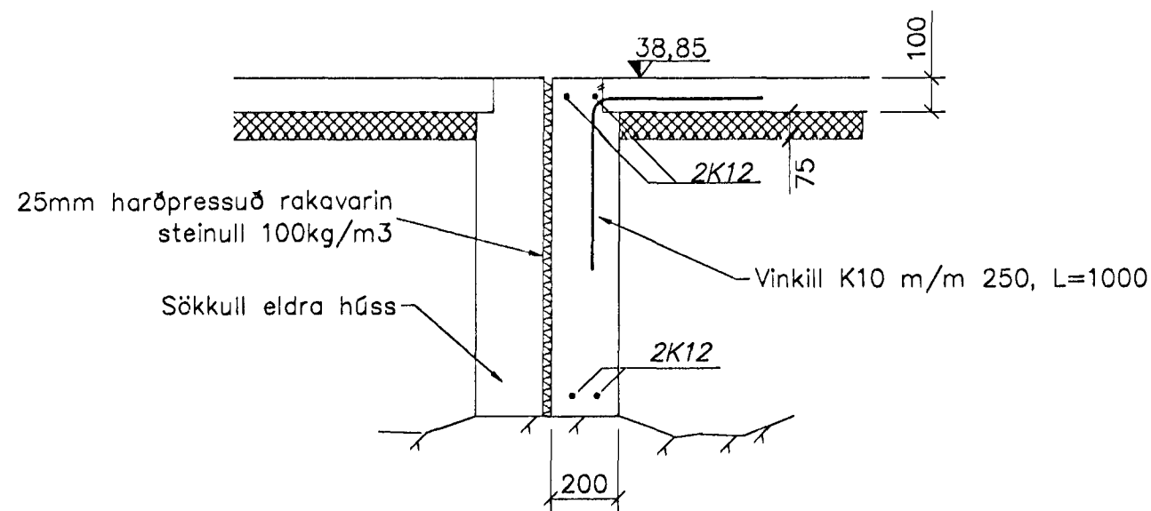
Snið C, 1:20
